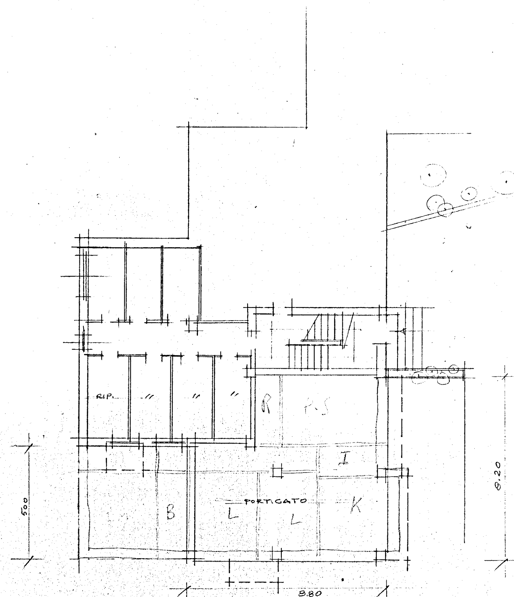
SITUAZIONE ATTUALE DEL P. TERRA
