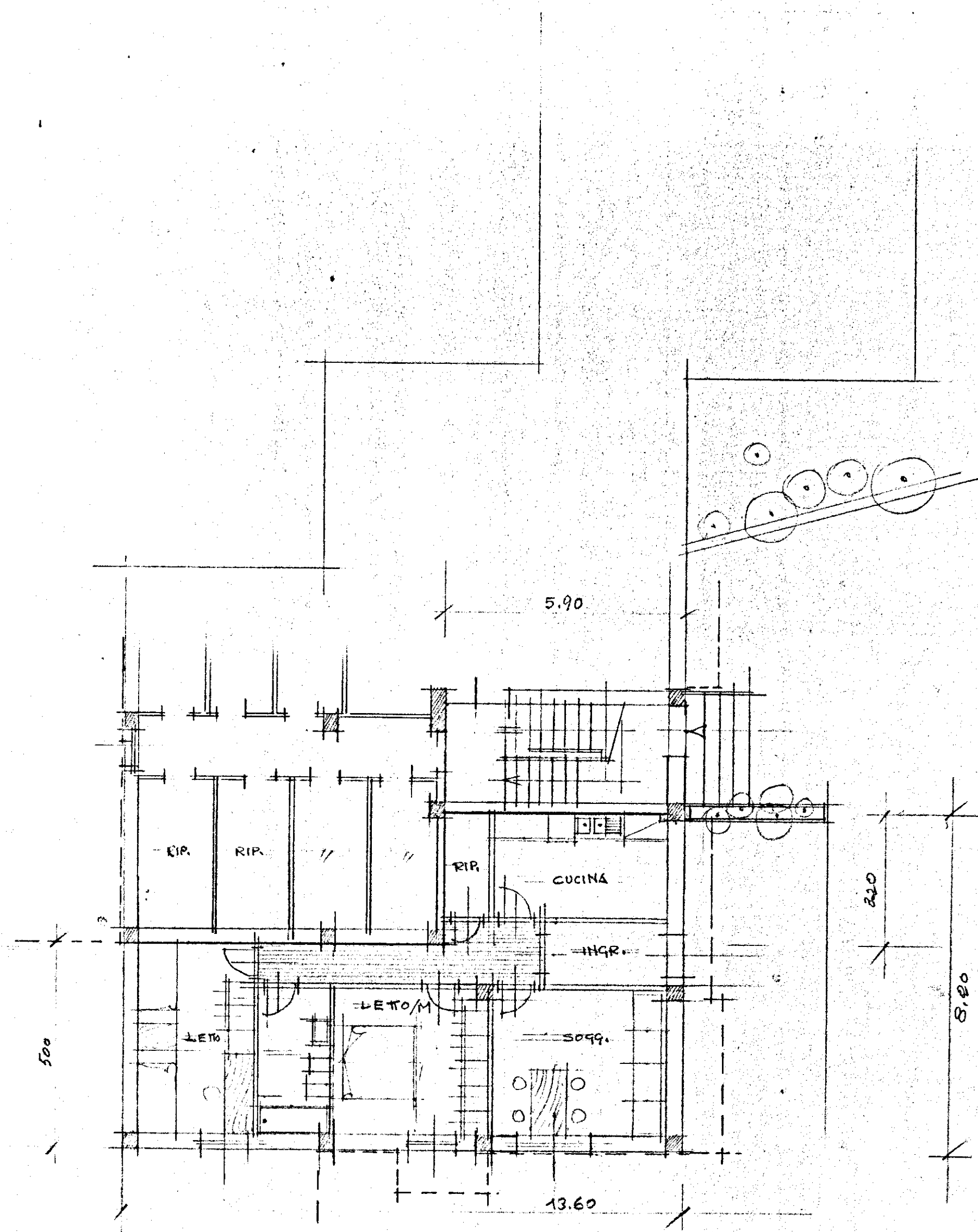
VARIANTE DEL PIANO TERRA DA PORTICO AD APPARTAMENTO
