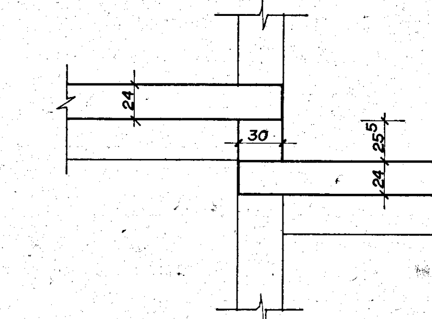
SEZ. G SOVRAPP. SOLAI DI 30 cm
