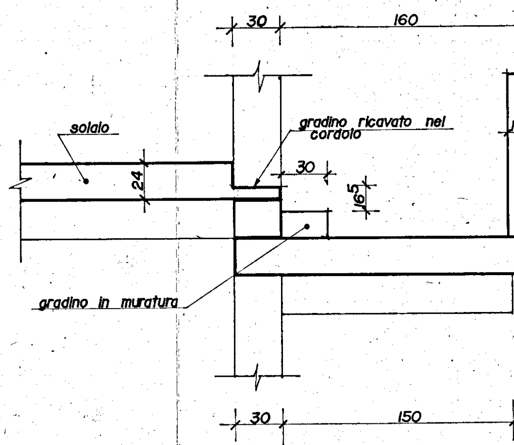
SEZ. B INGRESSO ALLOGGI
