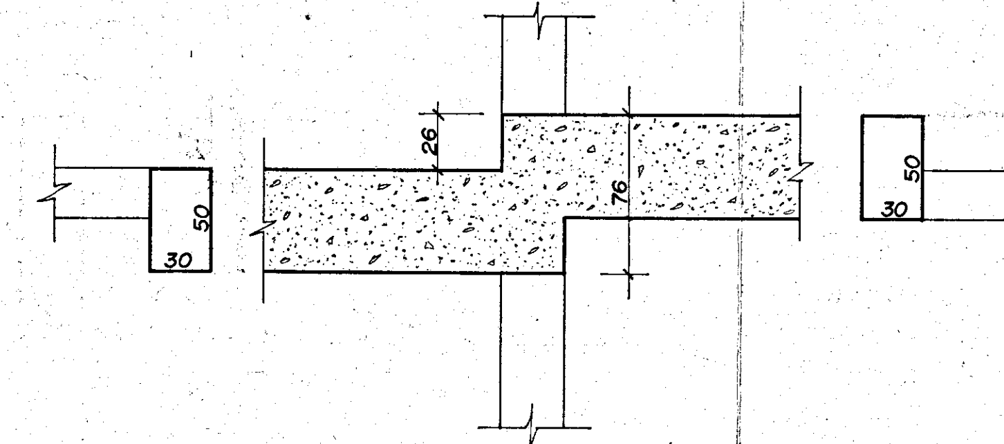
SEZ. E MENSOLA EXTRADOSSATA
