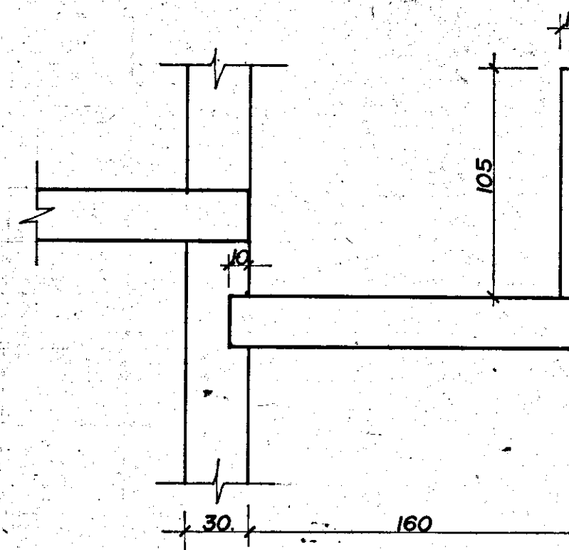
SEZ. H SOVRAPP. SOLAI 10 cm
