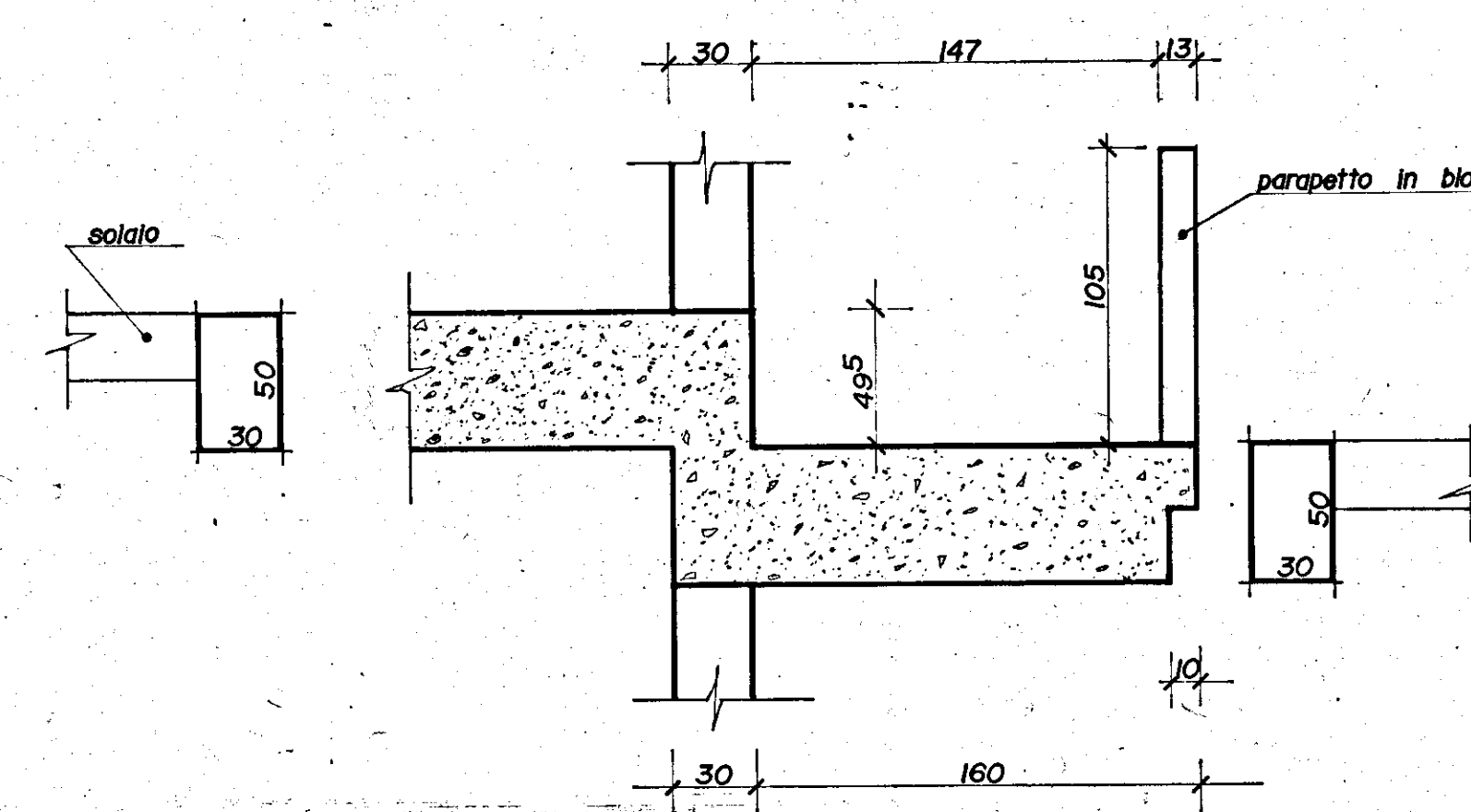
SEZ. A MENSOLA TIPO
