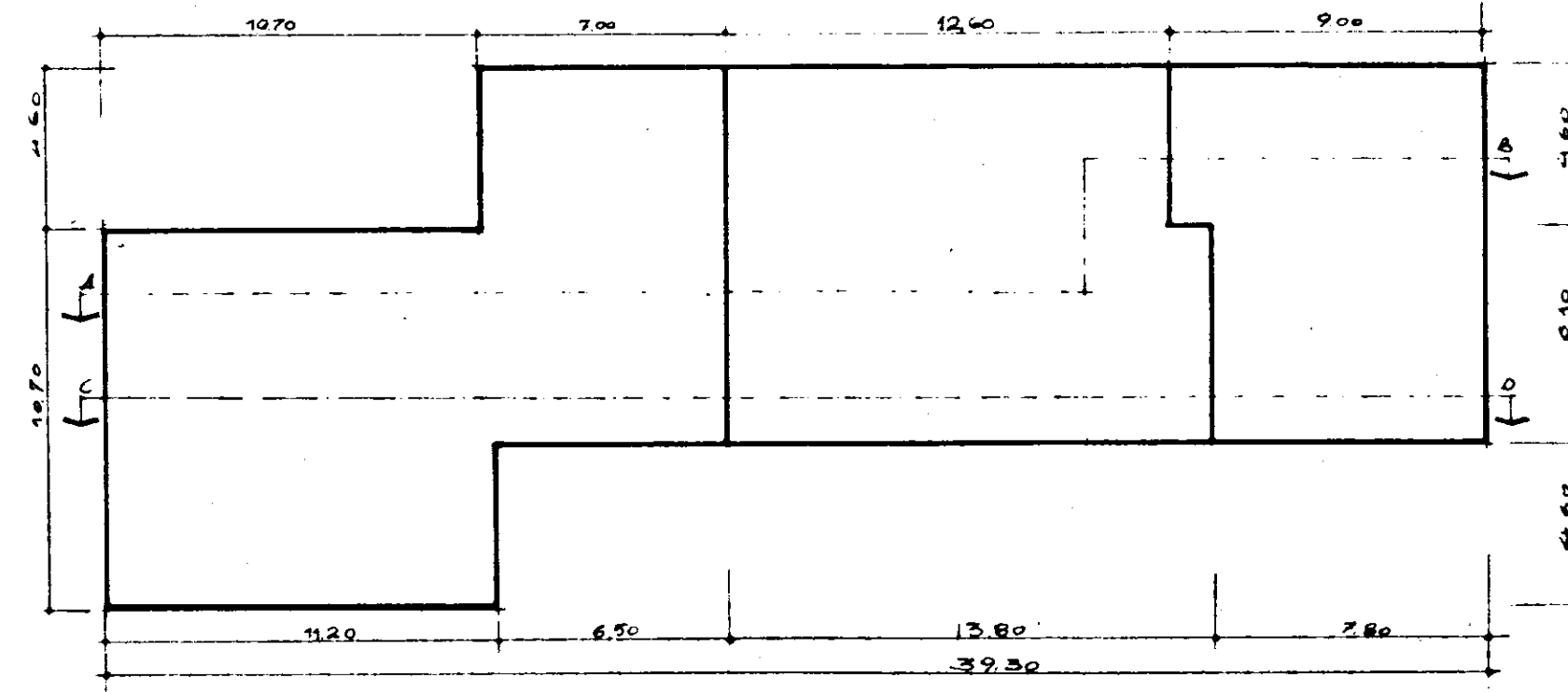
PIANTA MURATURE
