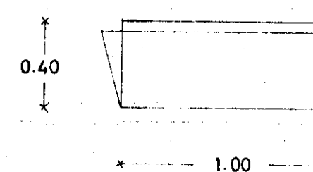
SERR. VASISTAS VERSO L'INTERNO A DUE ANTE N.32
