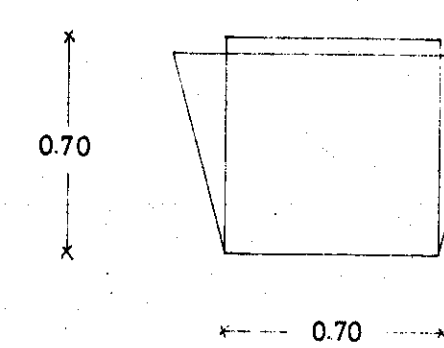
SERR. VASISTAS VERSO L'INTERNO N.31
