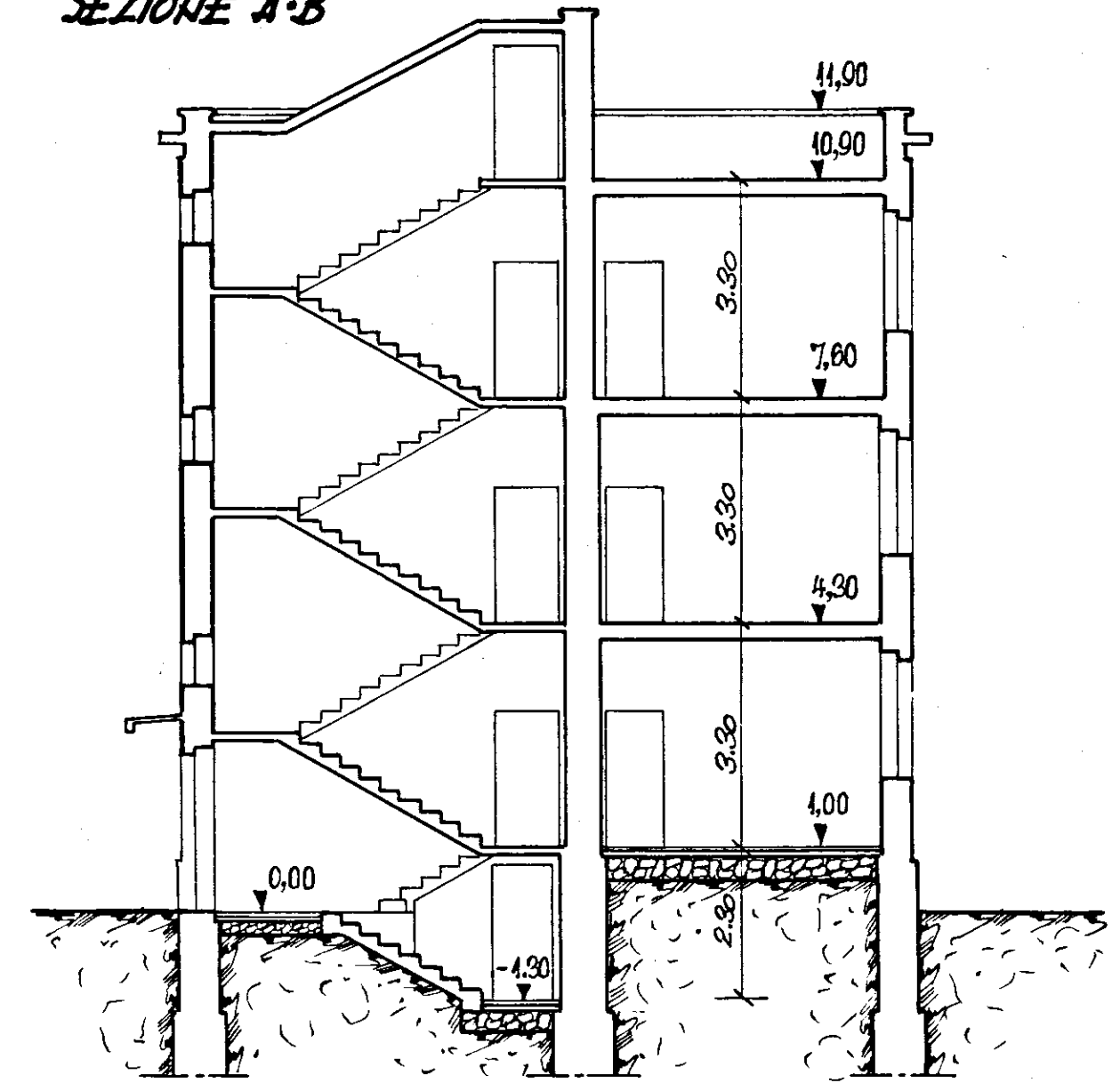
SEZIONE A-B
