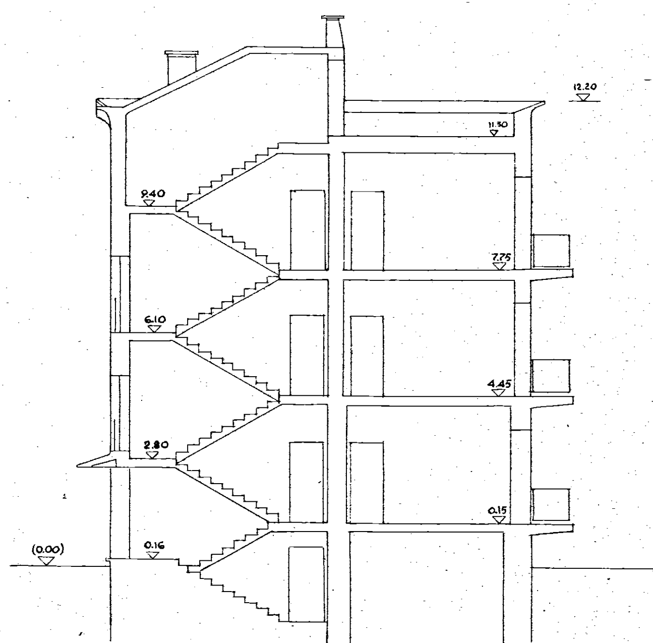
SEZIONE A-B
