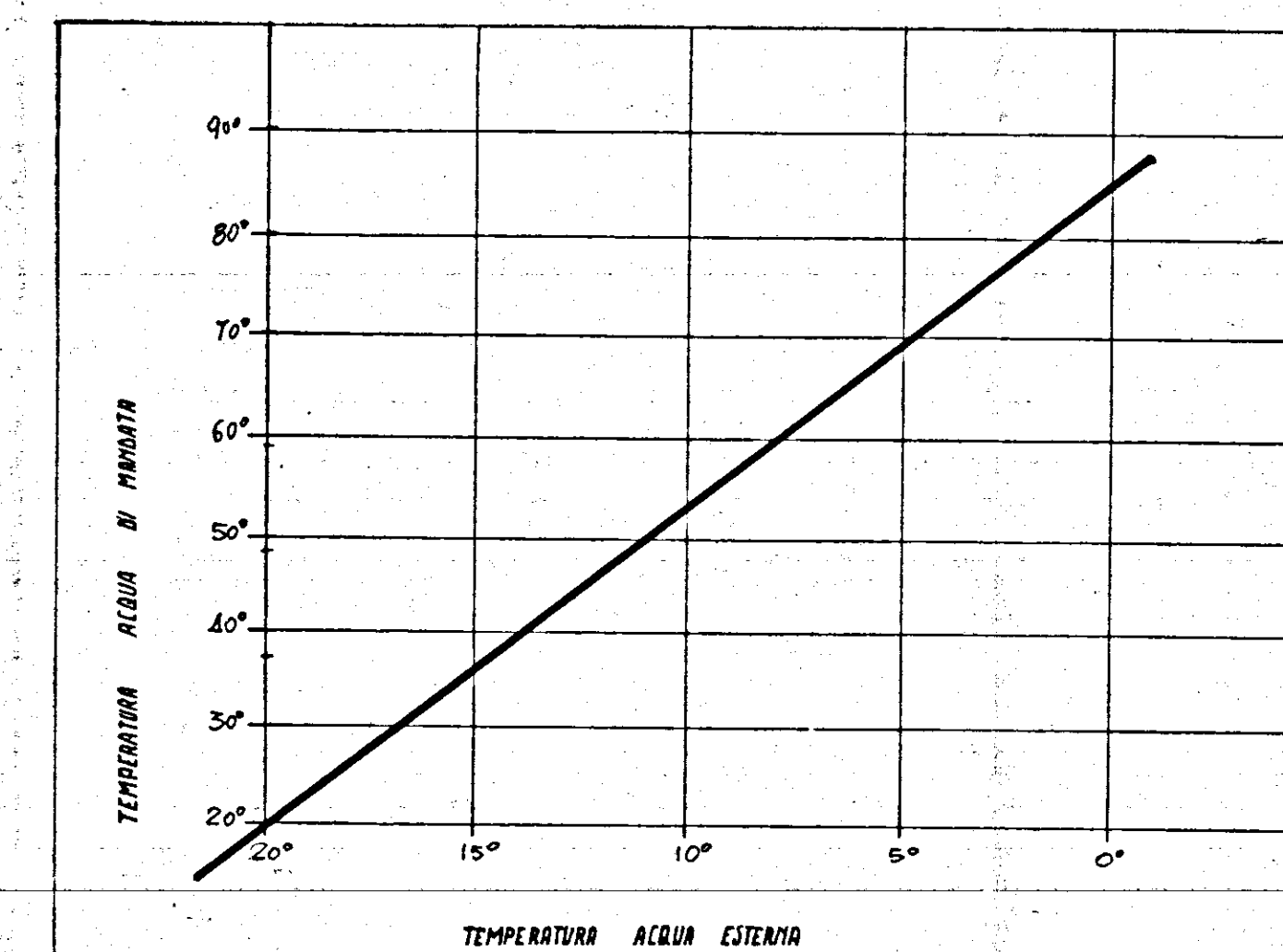
CURVA FUNZIONAMENTO IMPIANTO
