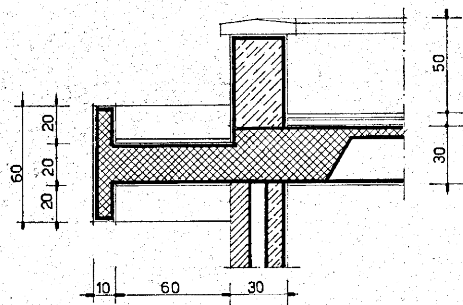
particolare A-A rapp. 1:20
