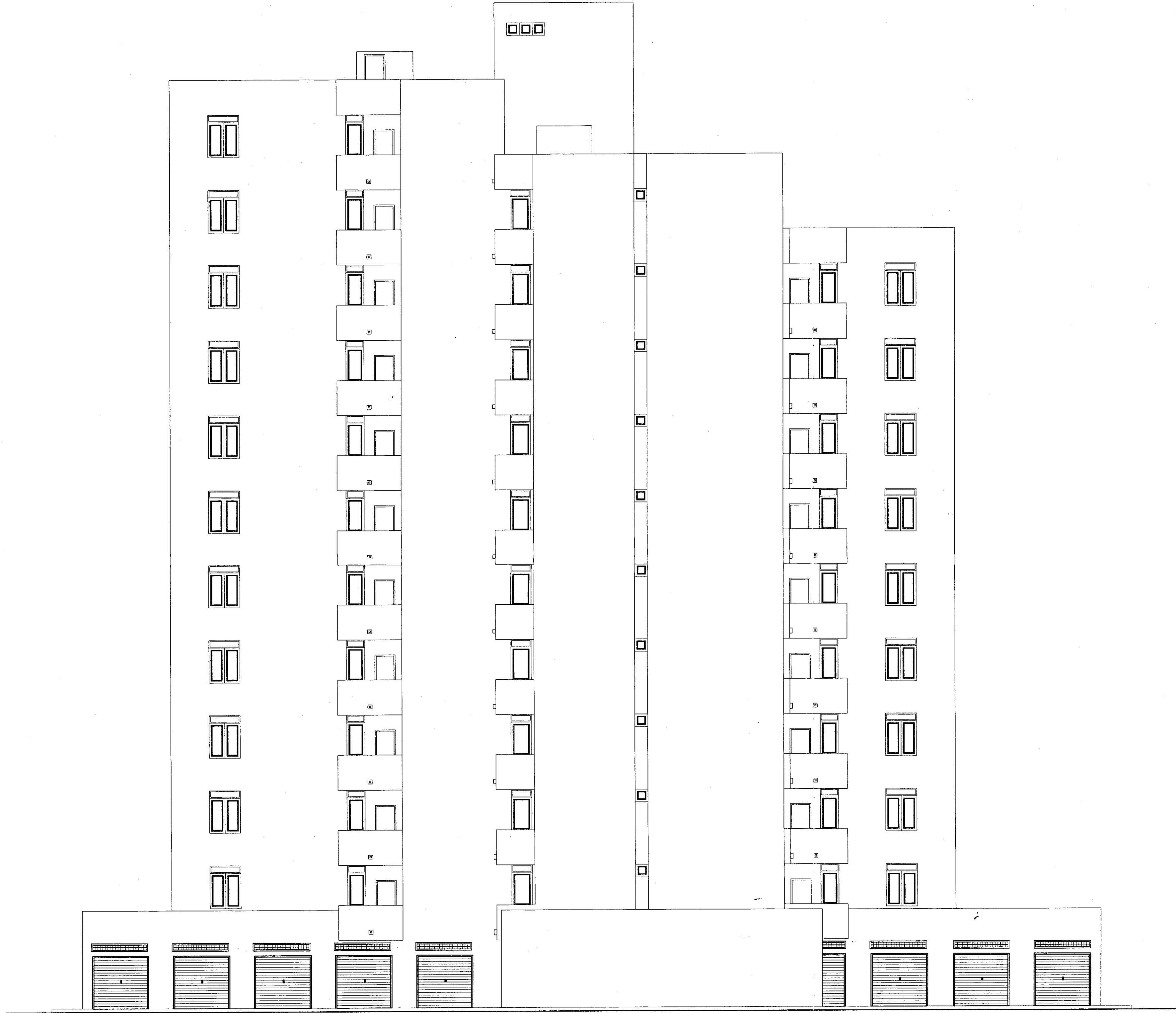
PROSPETTO - C -
