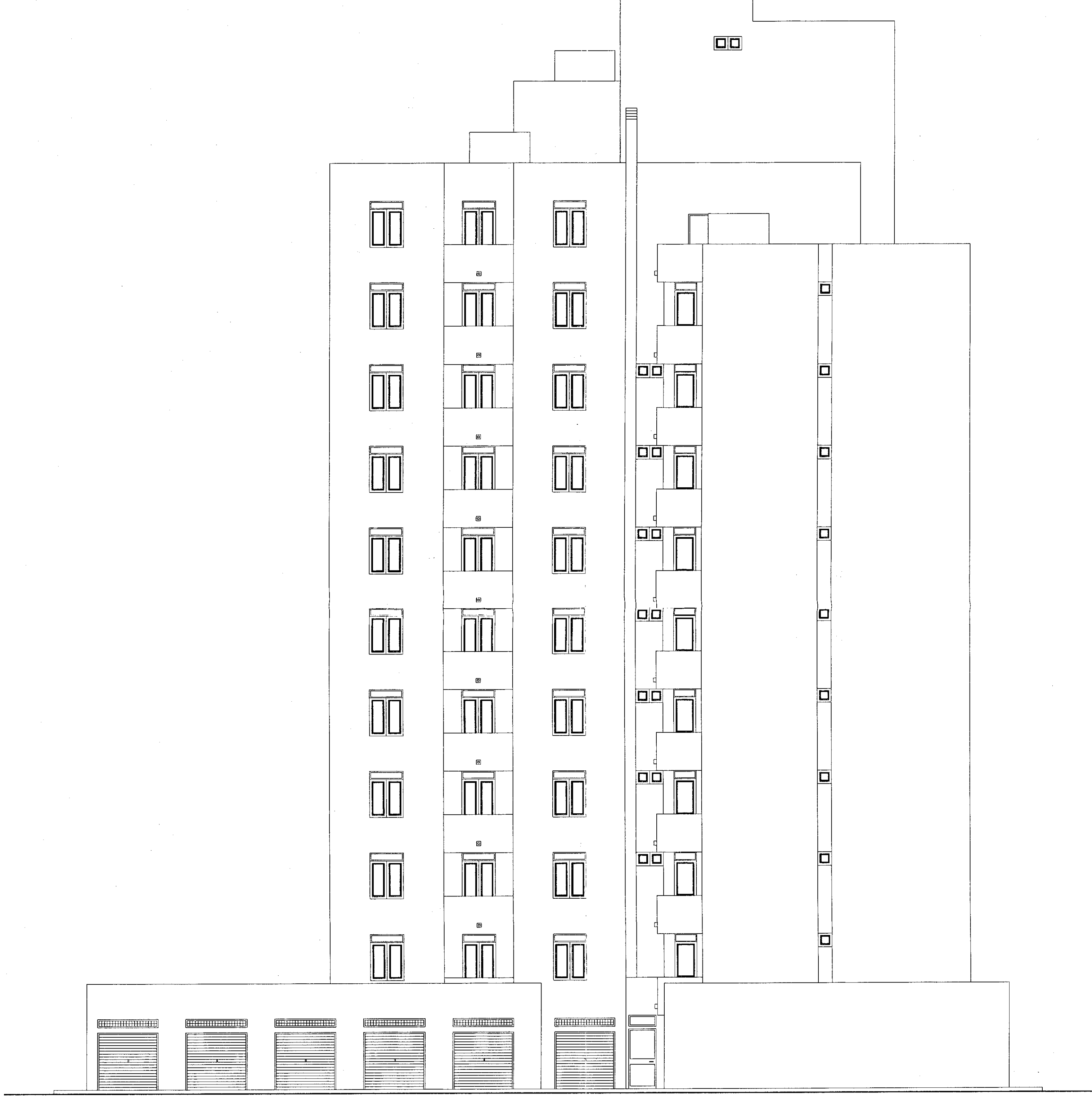
PROSPETTO - D -
