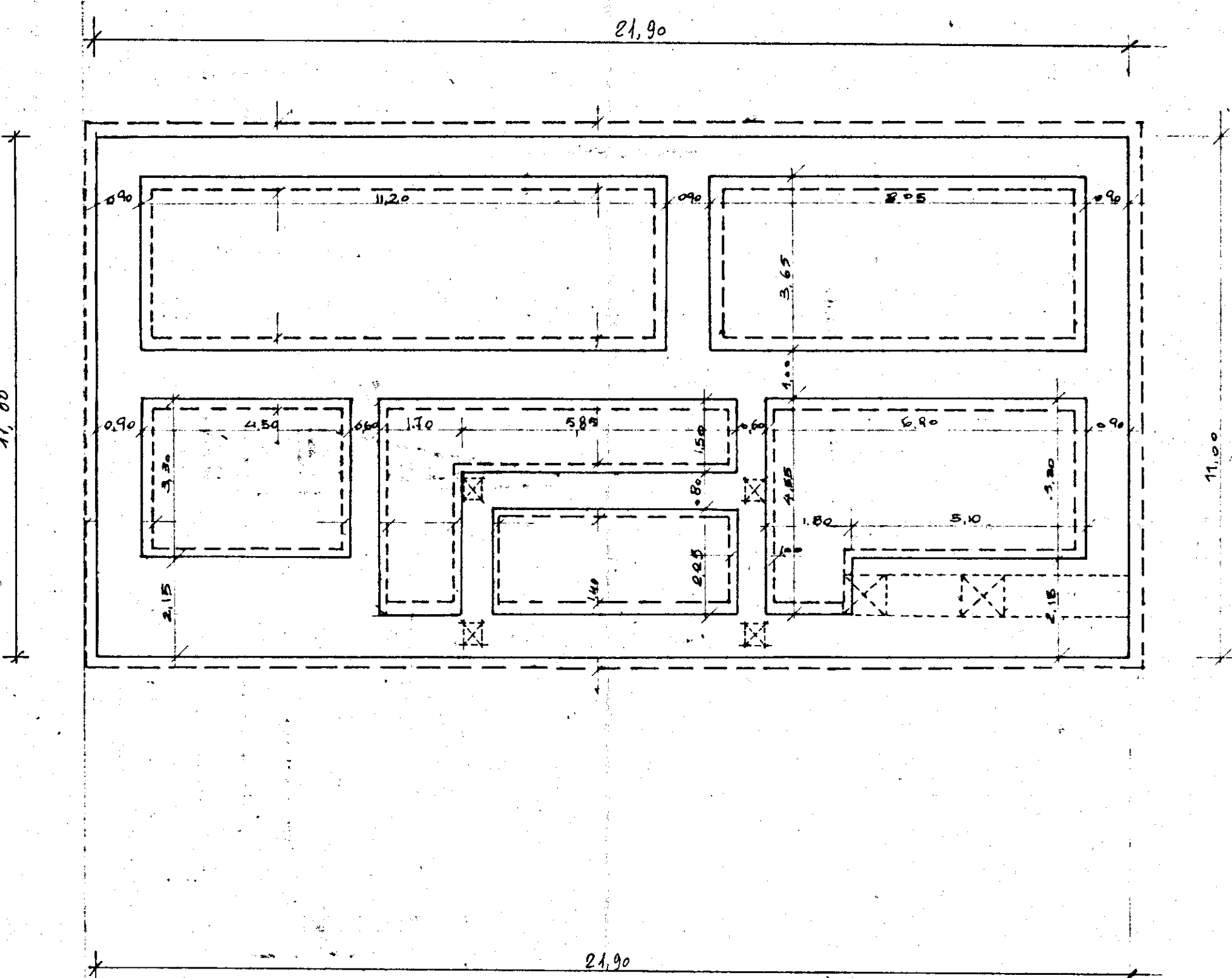
PIANTA FONDAZIONI
