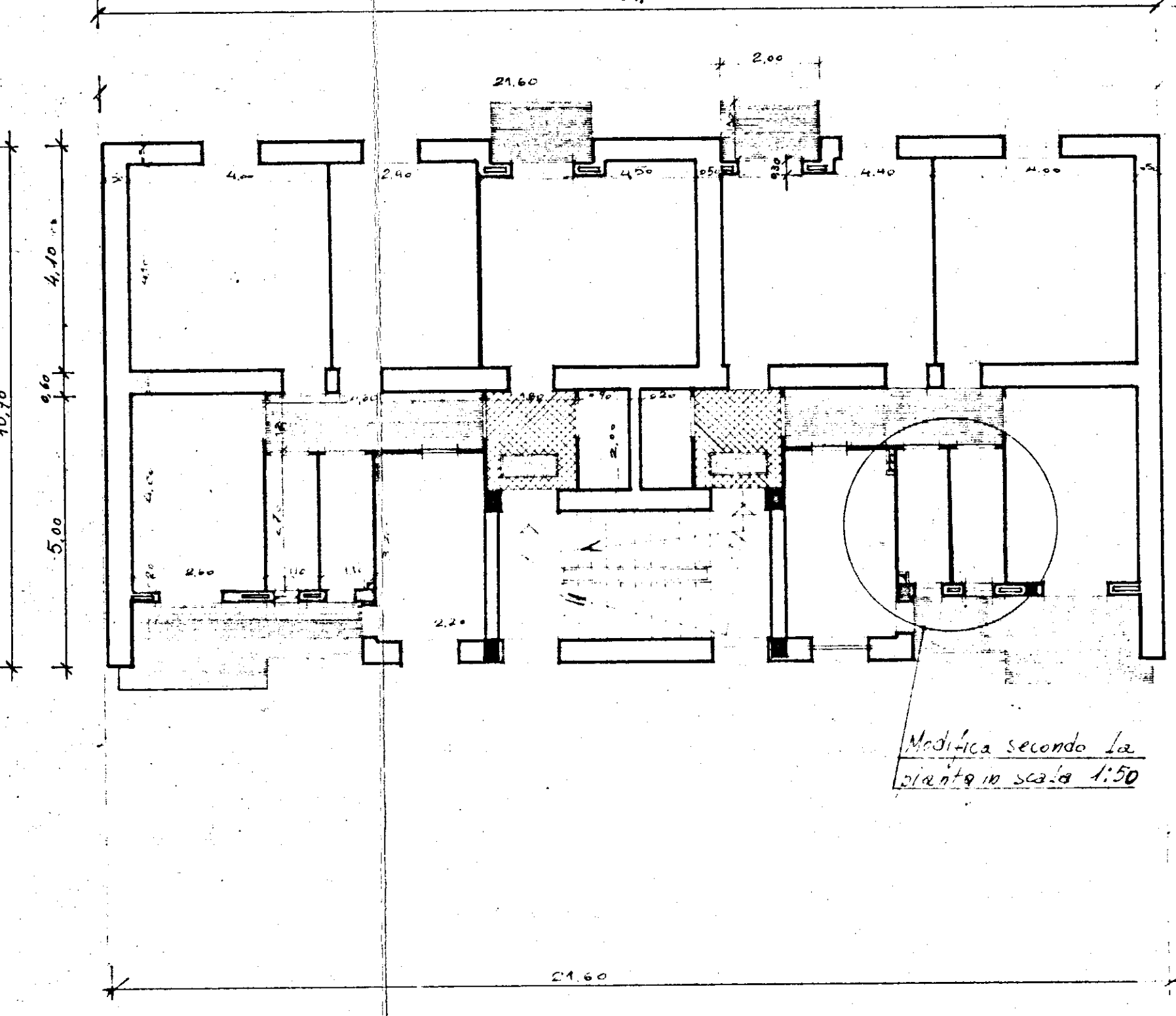
PRIMO PIANO
