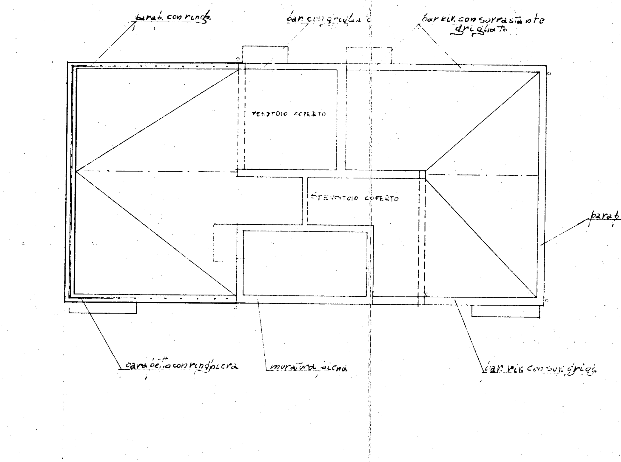
PIANTA TERRAZZA
