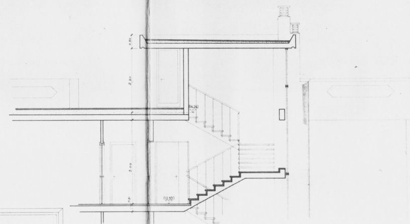
SEZIONE a - a particolare torrino scala
