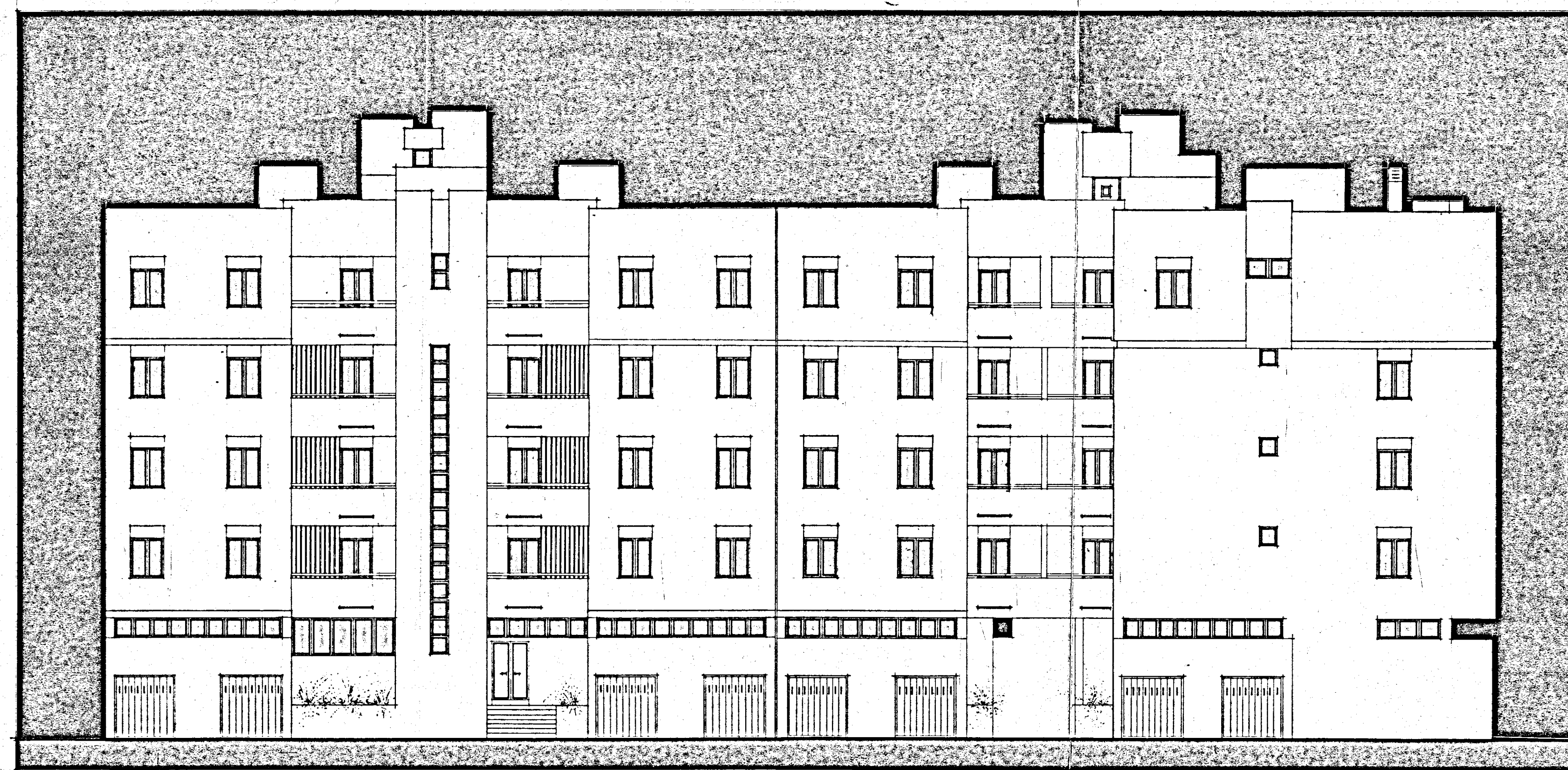
PROSPETTO -C-
