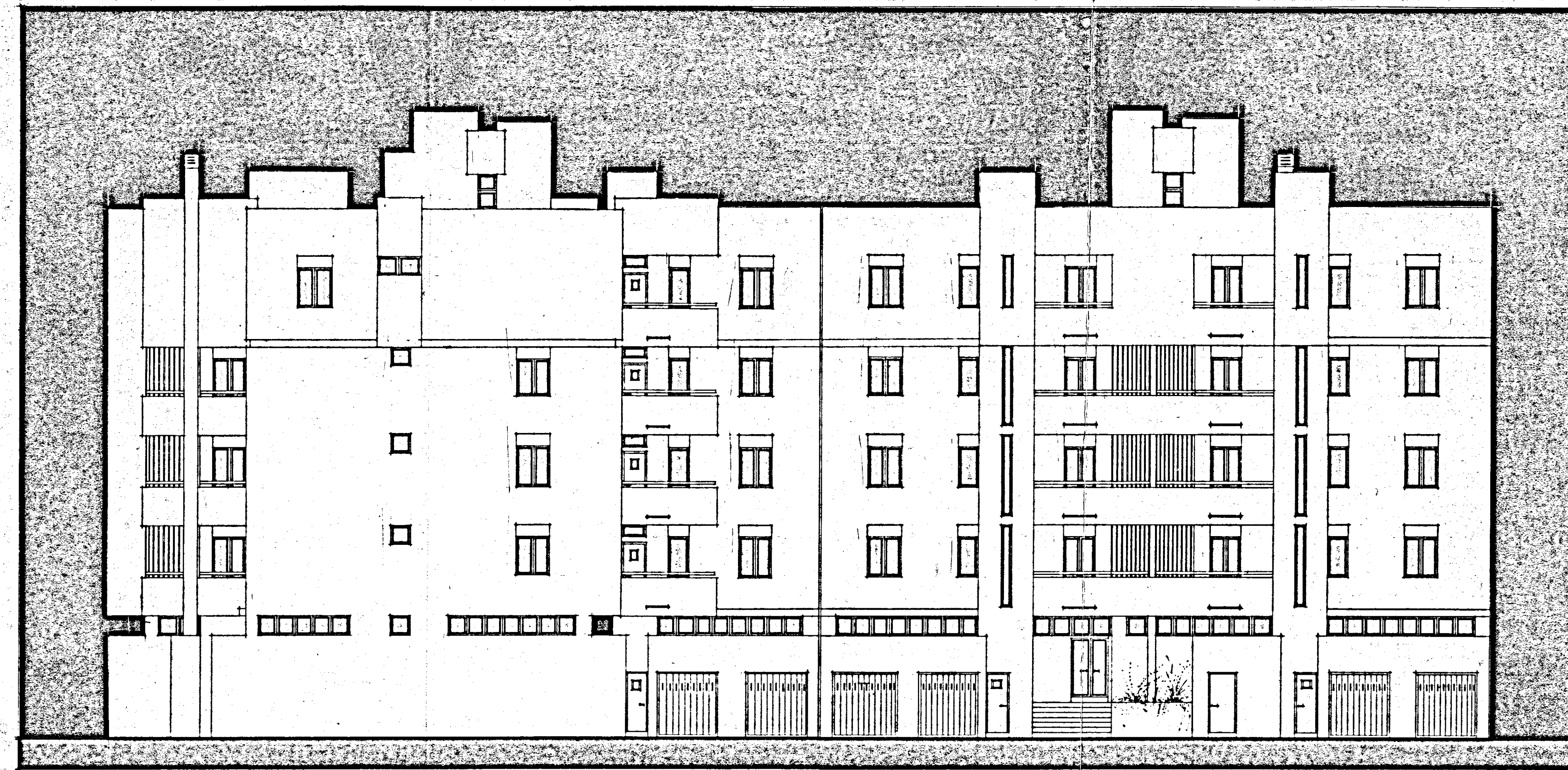
PROSPETTO -A-
