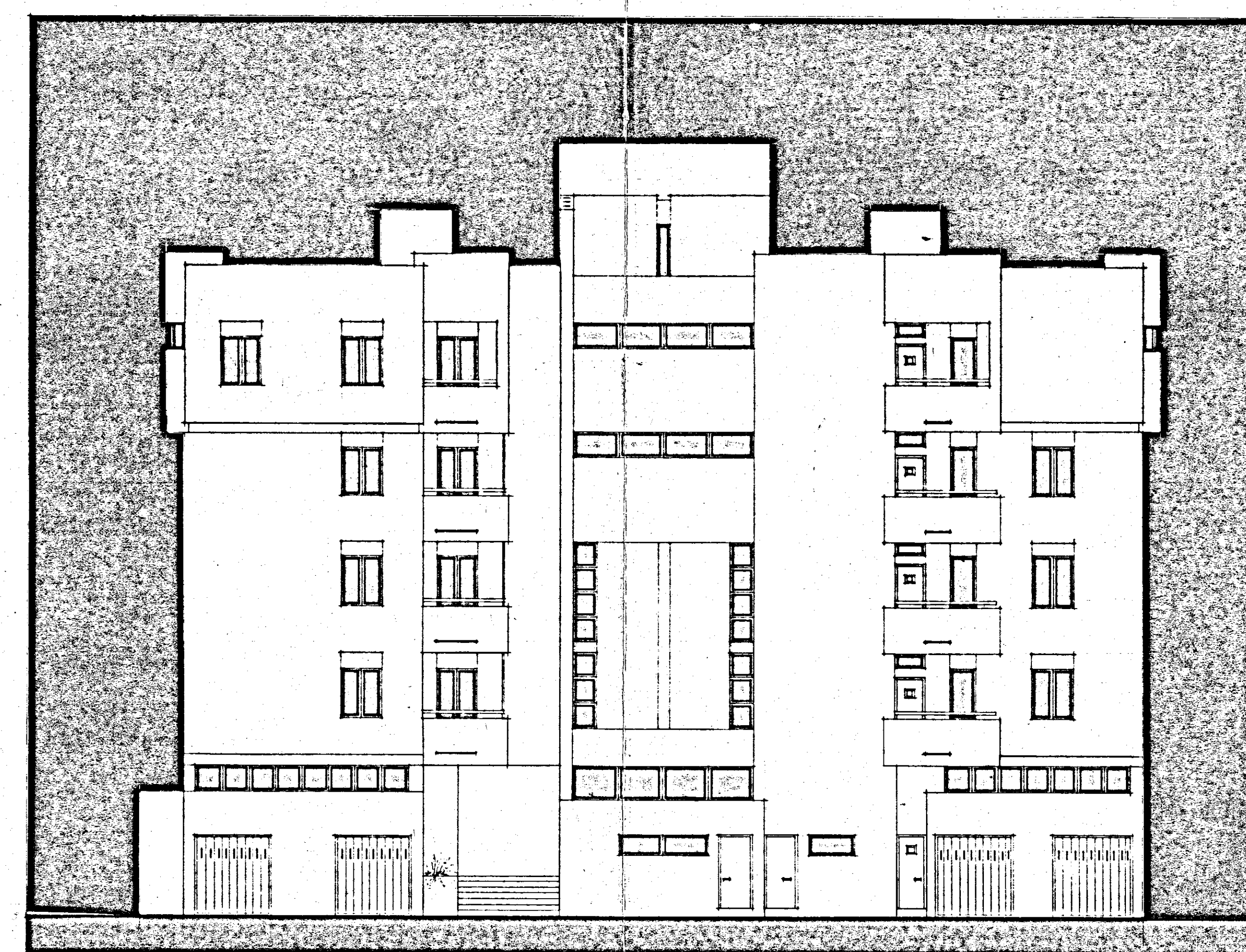
PROSPETTO -D-
