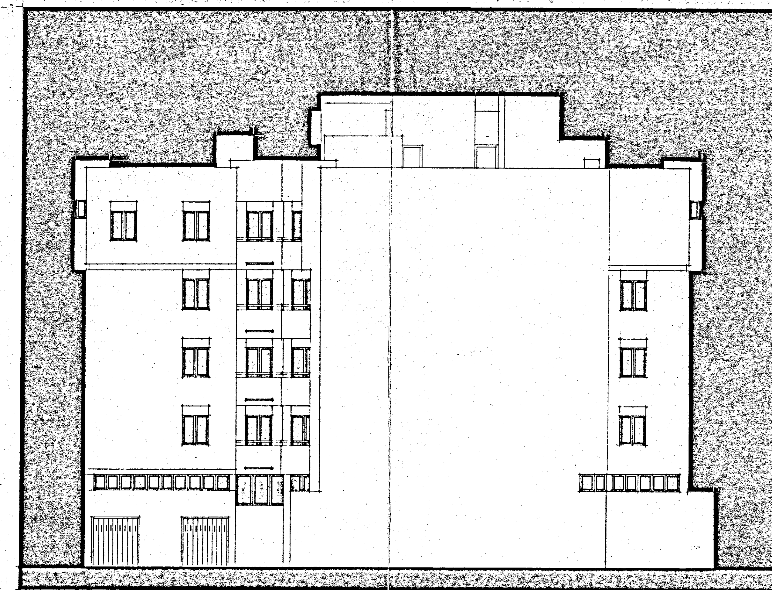
PROSPETTO -B-
