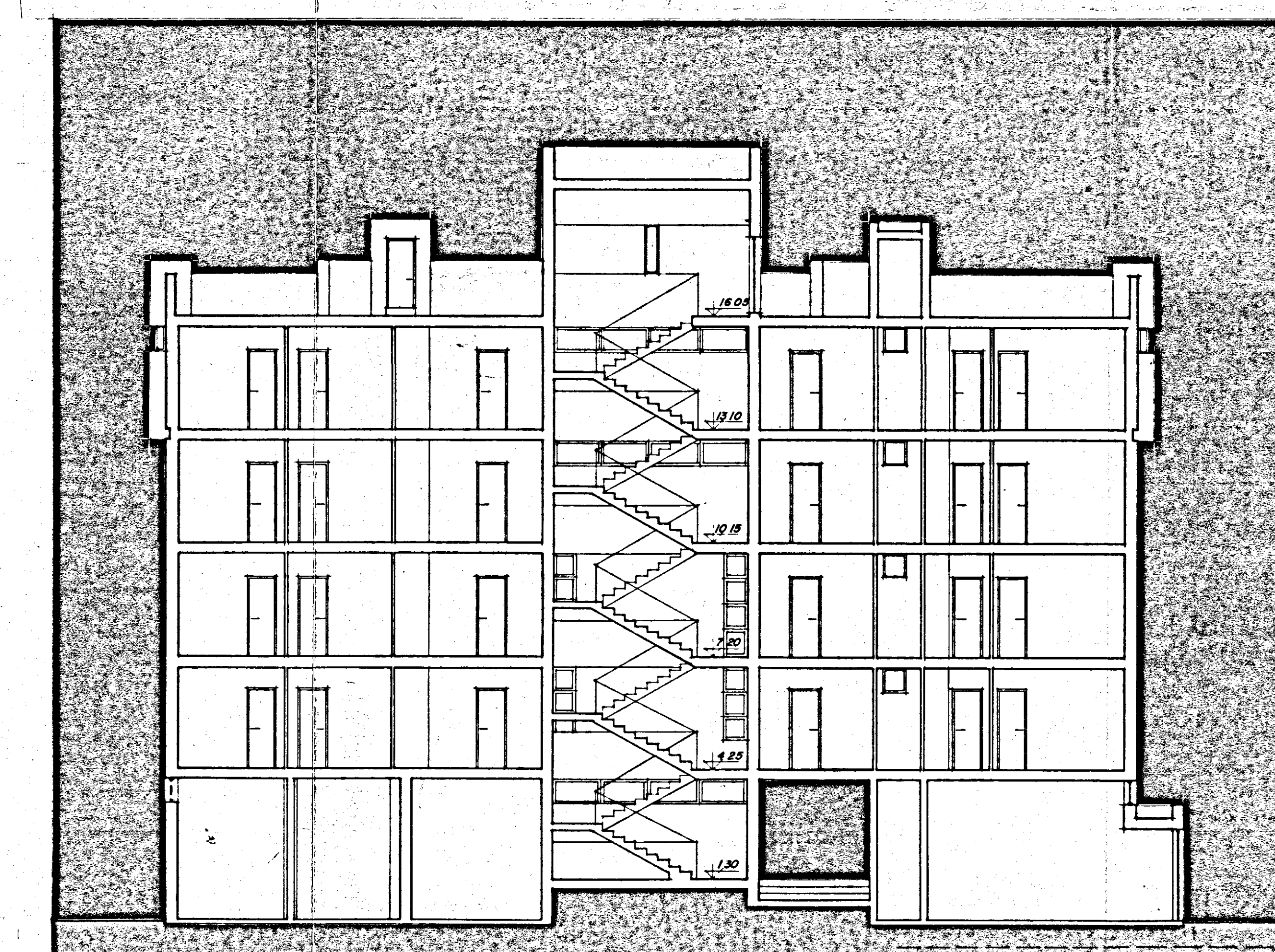
SEZIONE Y-Y
