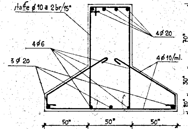
sez. trav. B-B
