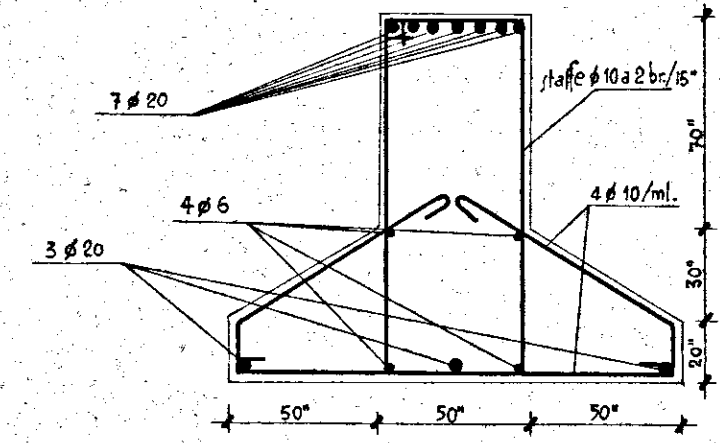
sez. trav. D-D
