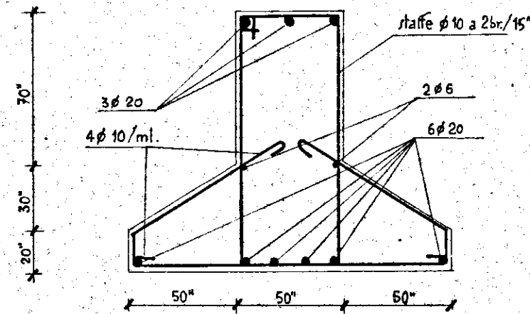
sez. trav. A-A
