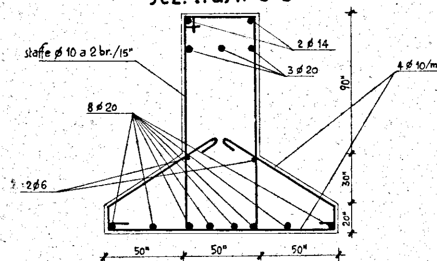
sez. trav. C-C
