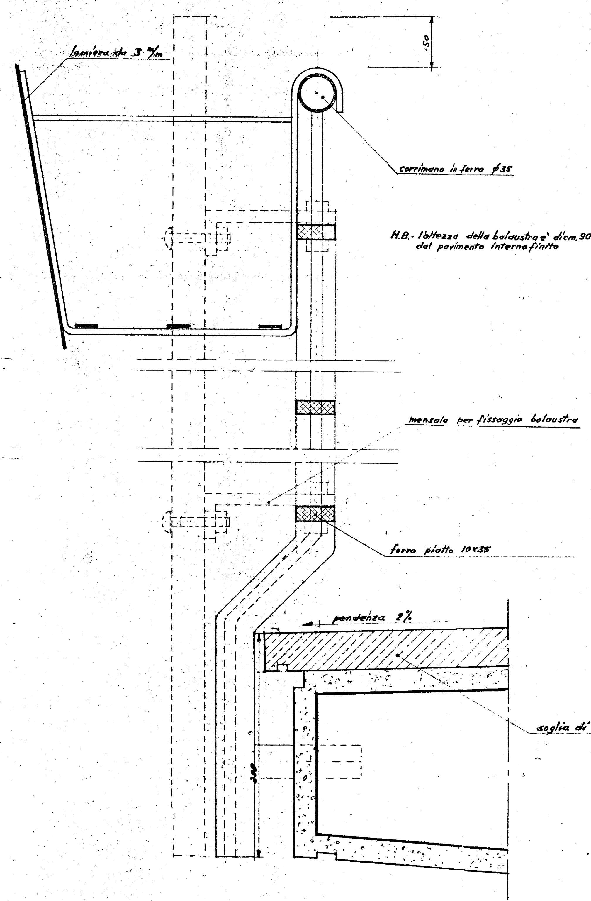
SEZIONE A-A
