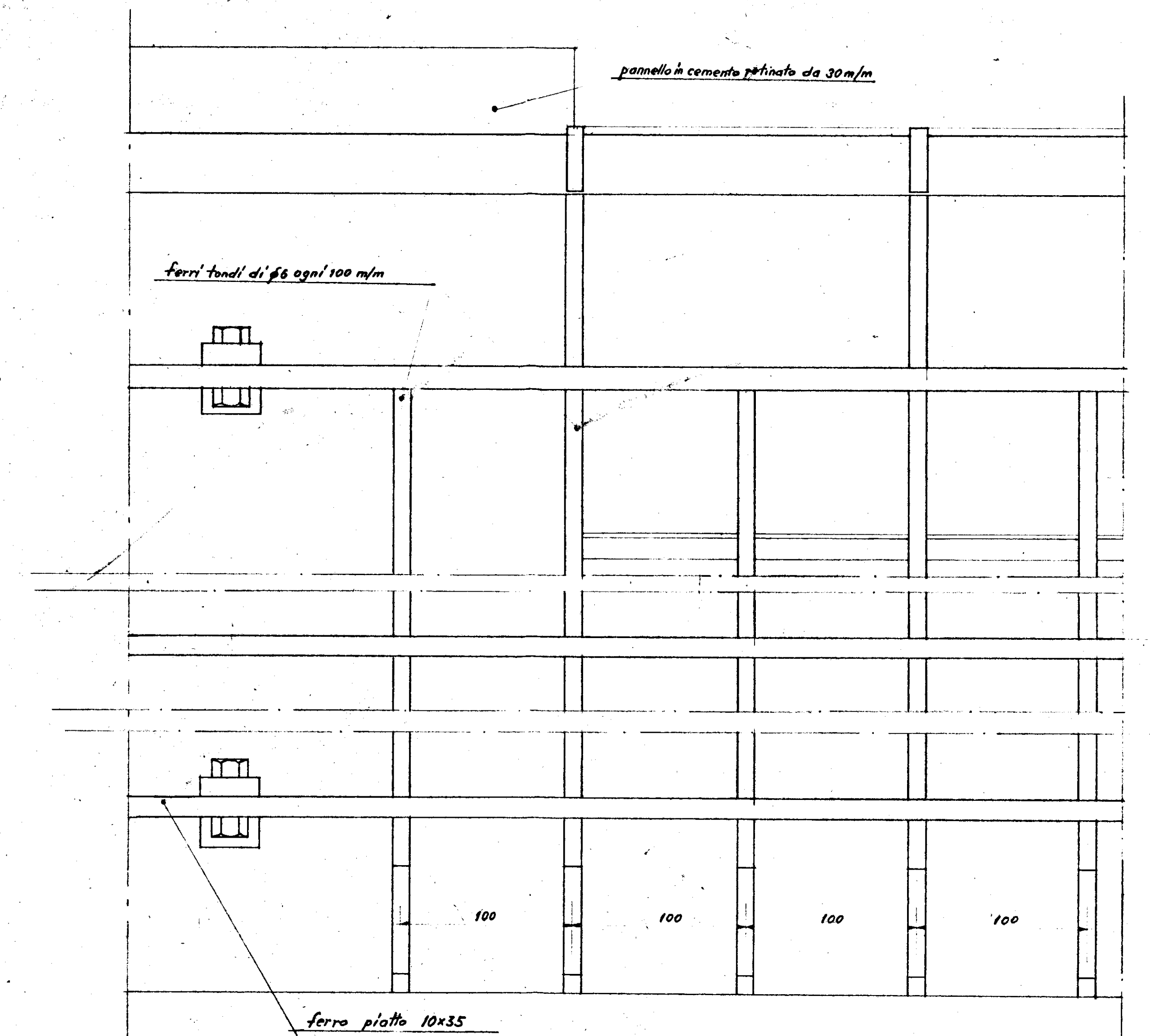
PROSPETTO INTERNO
