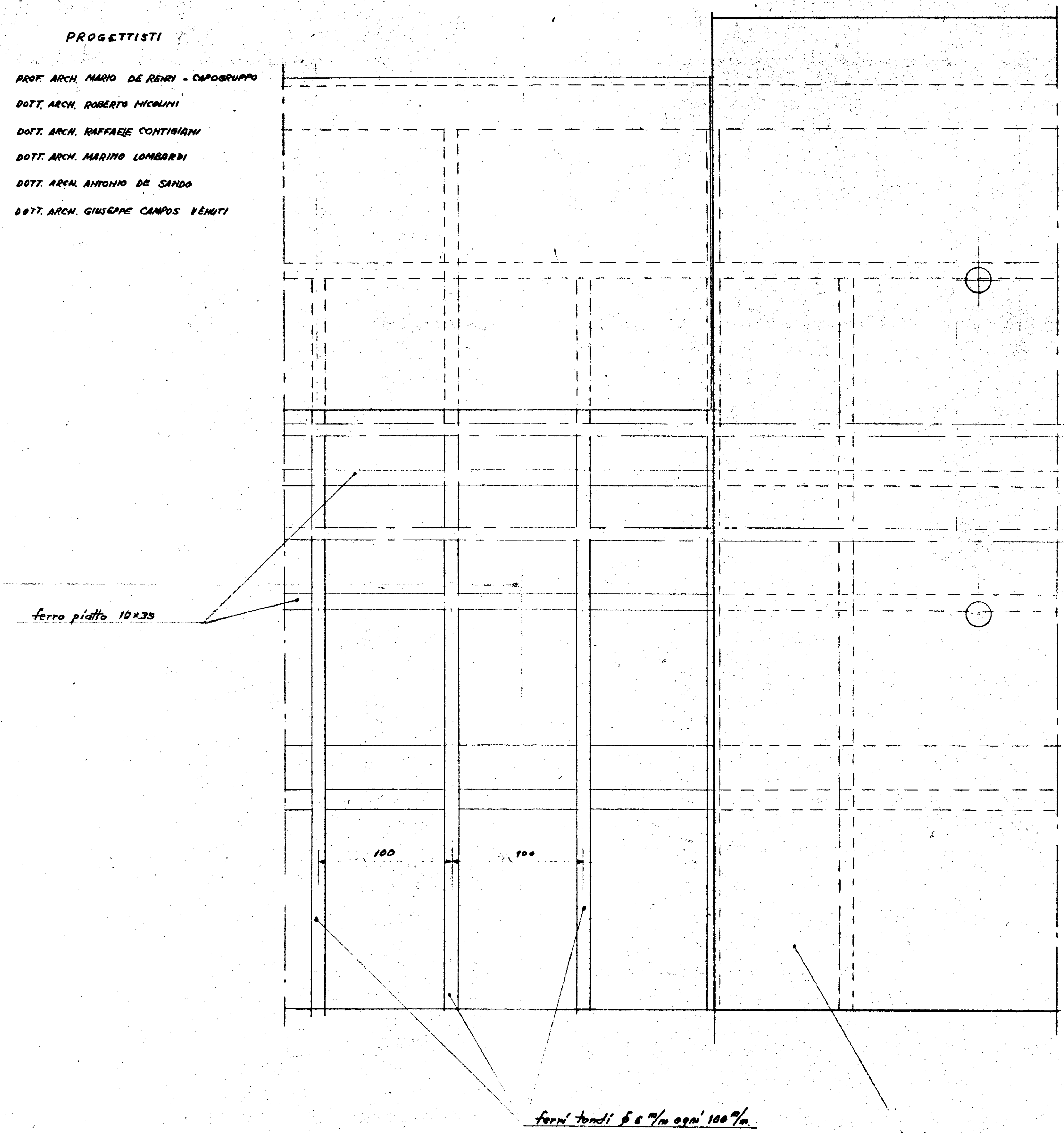
PROSPETTO ESTERNO
