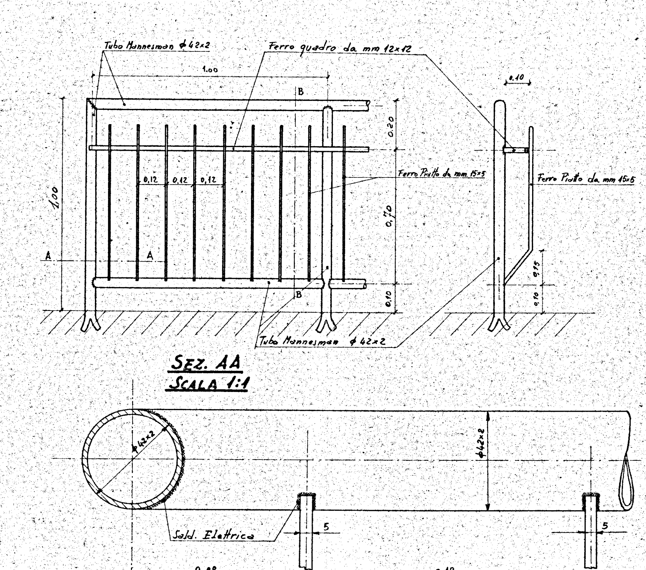
RINGHIERA PER BALCONI E VERANDE SCALA 1:10
