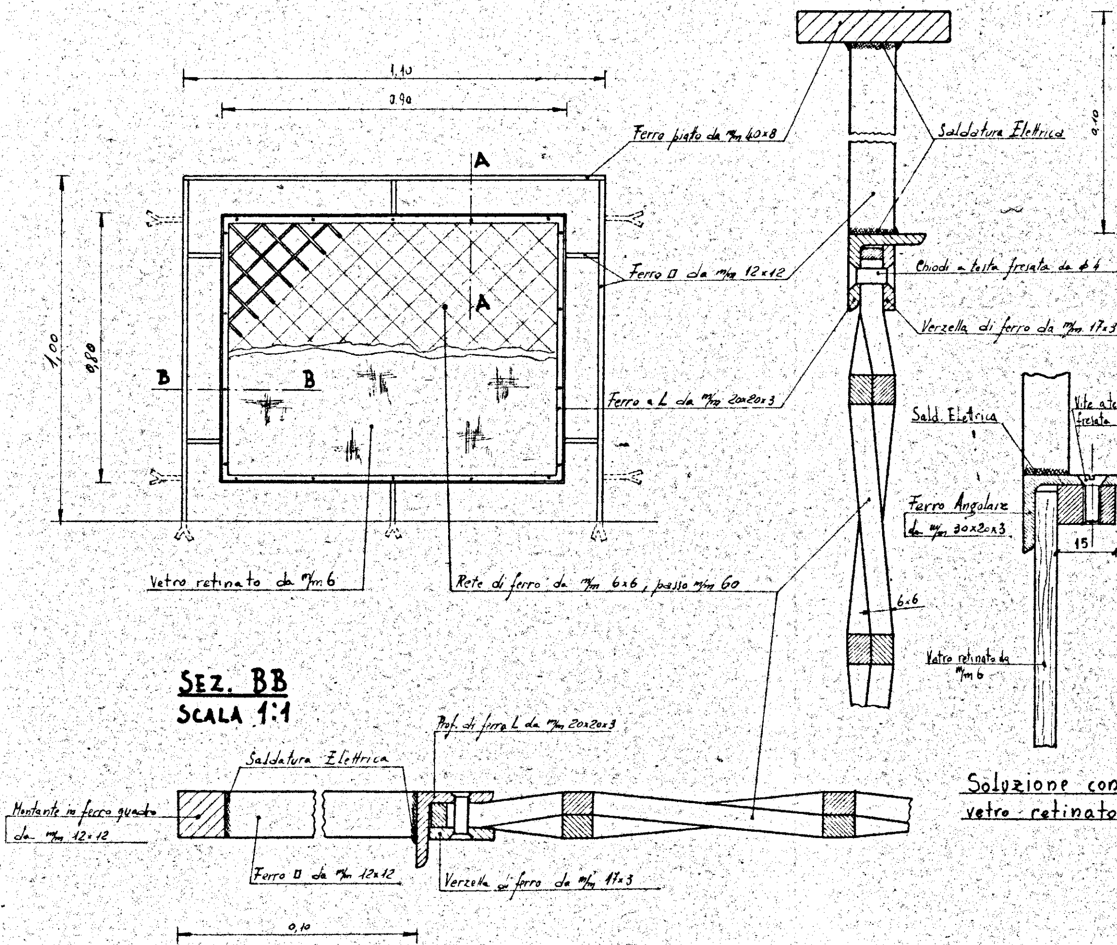
RINGHIERA PER BALCONI E VERANDE SCALA 1:10
