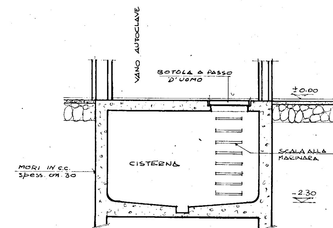
SEZIONE FATTA SUL VANO AUTOCLAVE RAPP. 1:50
