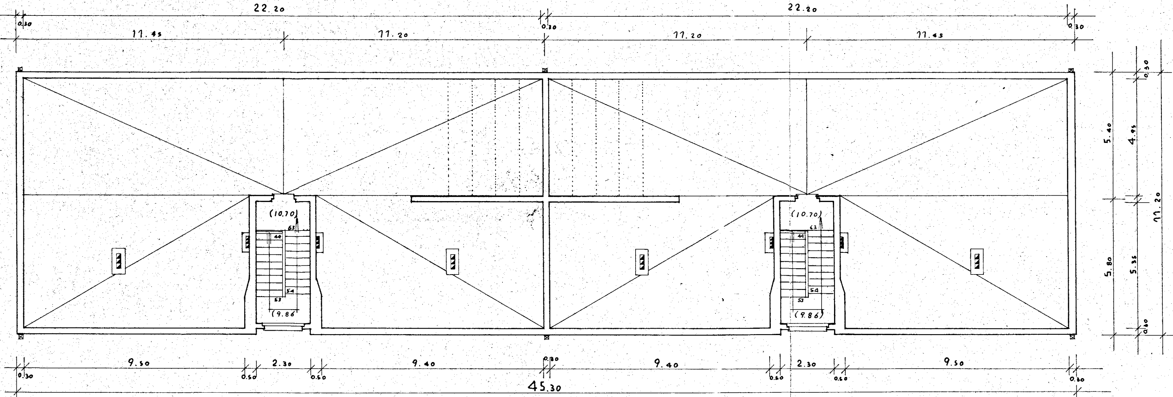
DIS. 45 PIANTA PIANO COPERTURA RAPP. 1:100
