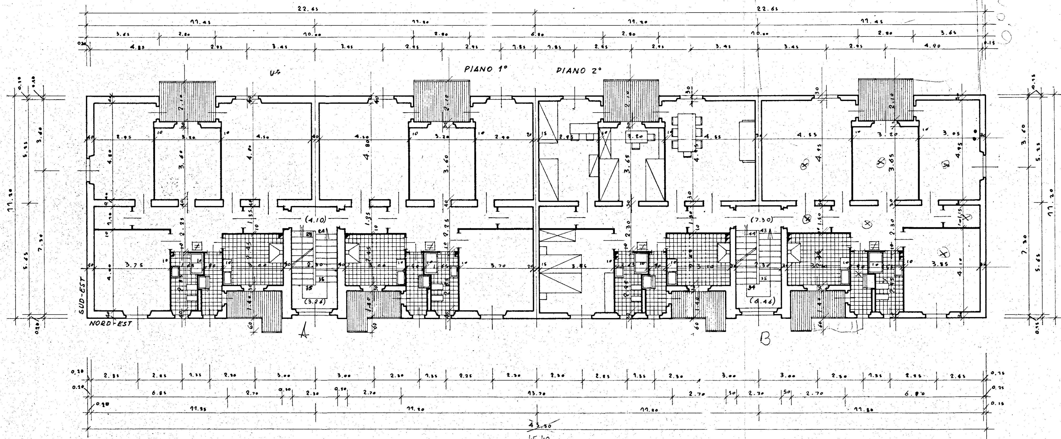
DIS. 44 PIANTA PIANO 1° E 2° RAPP. 1:100
