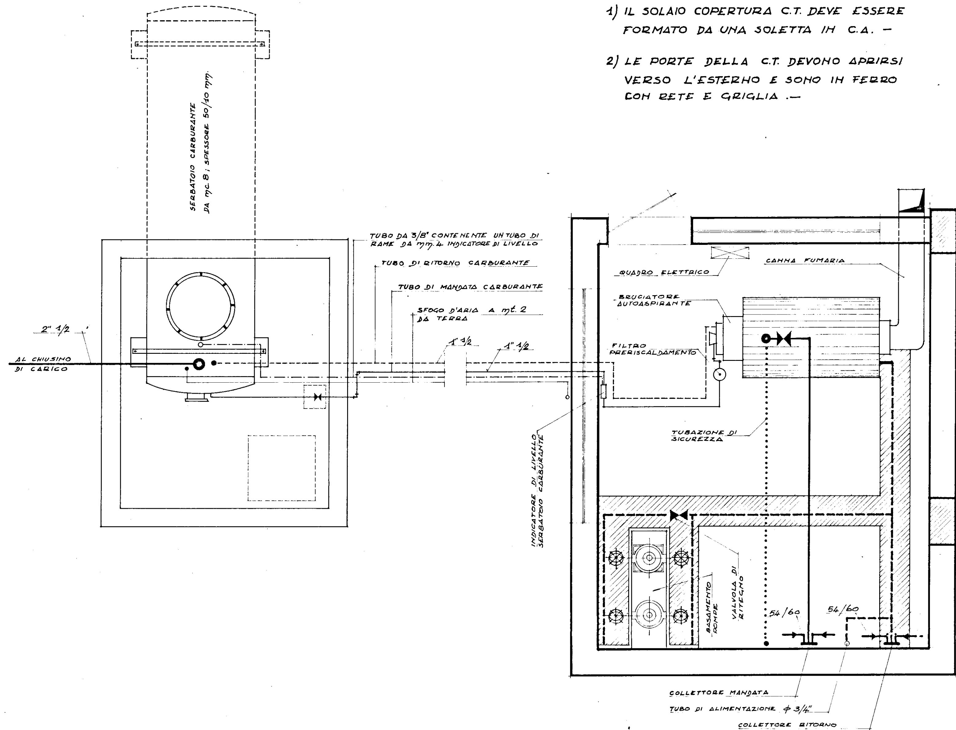
pianta della centrale termica - rapp. 1/25
