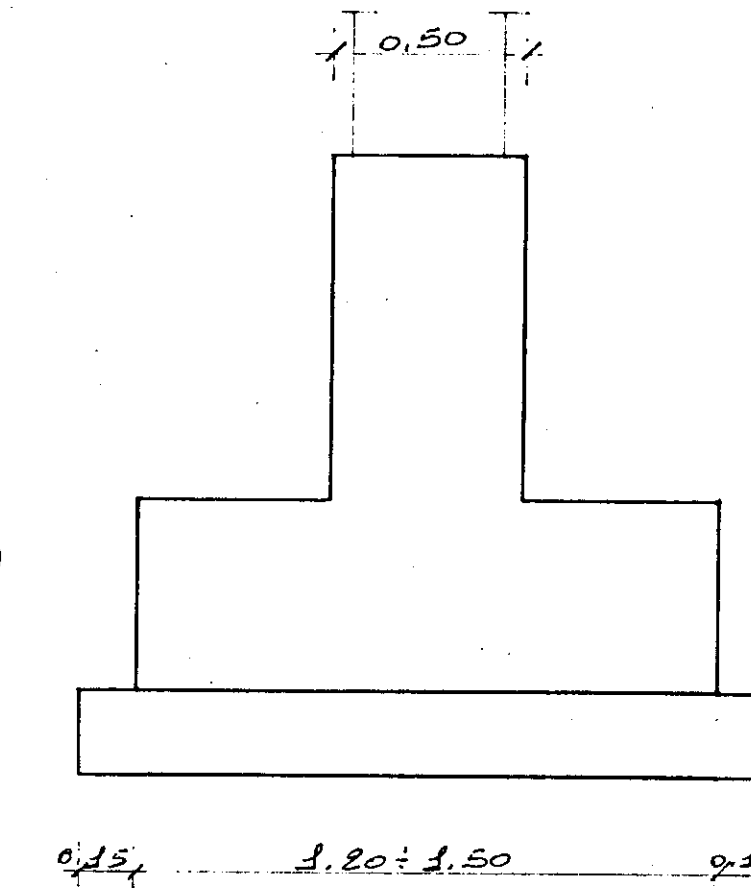
Sezione tipo travi orizzontali
