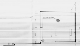
SEZIONE A-B
