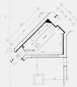
PIANTA CENTRALE-TERMICA (scale 1:50)
