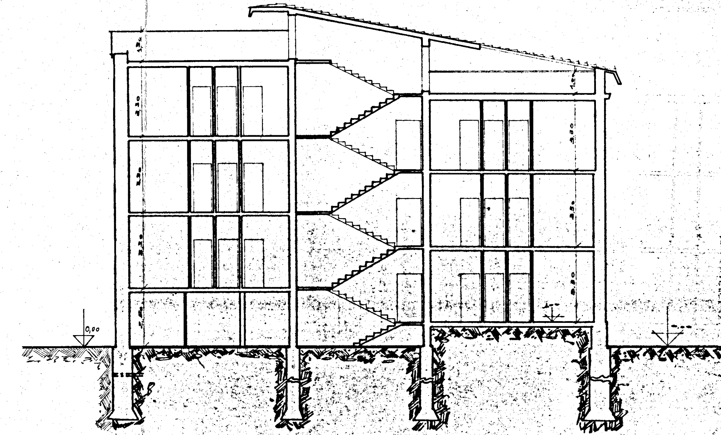
SEZIONE LONGITUDINALE
