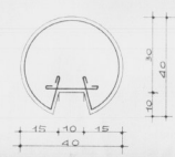
SEZIONE PILASTRI
