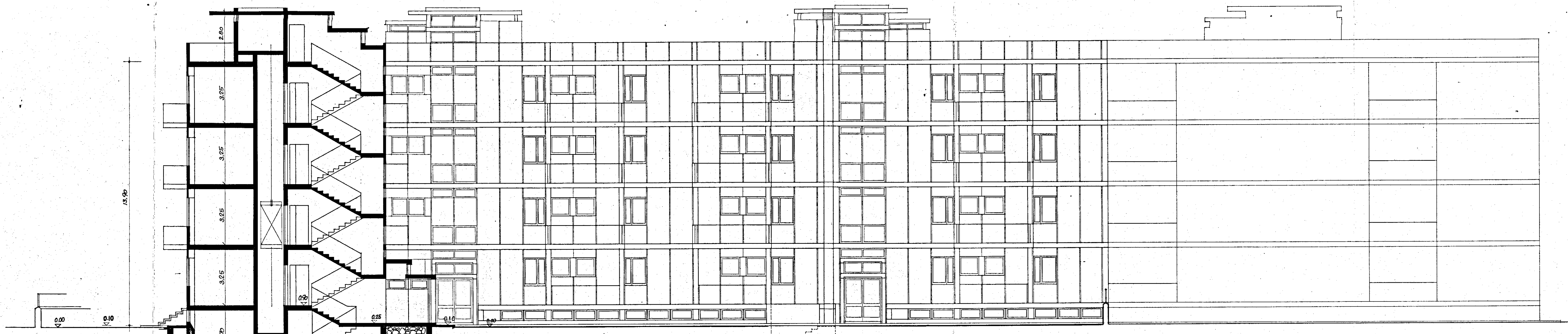
PROSPETTO-SEZIONE NORD - RAPP. 1:100
