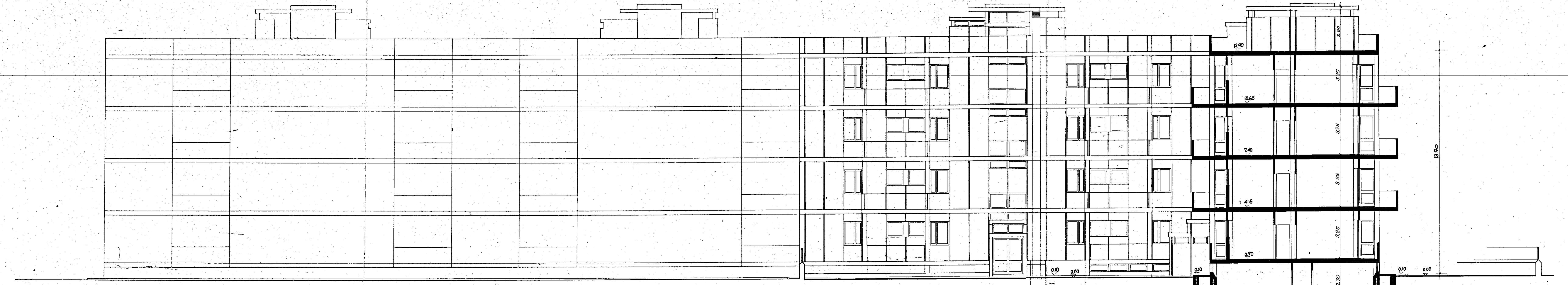
PROSPETTO-SEZIONE OVEST - RAPP. 1:100
