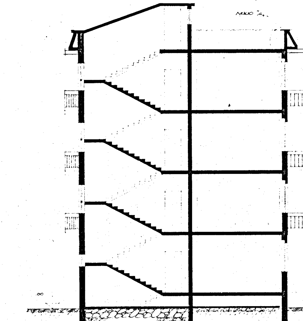
SEZIONE X-X
