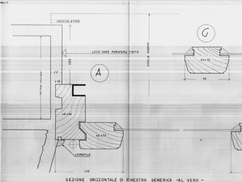
SEZIONE ORIZZONTALE DI FINESTRA GENERICA -AL VERO -
