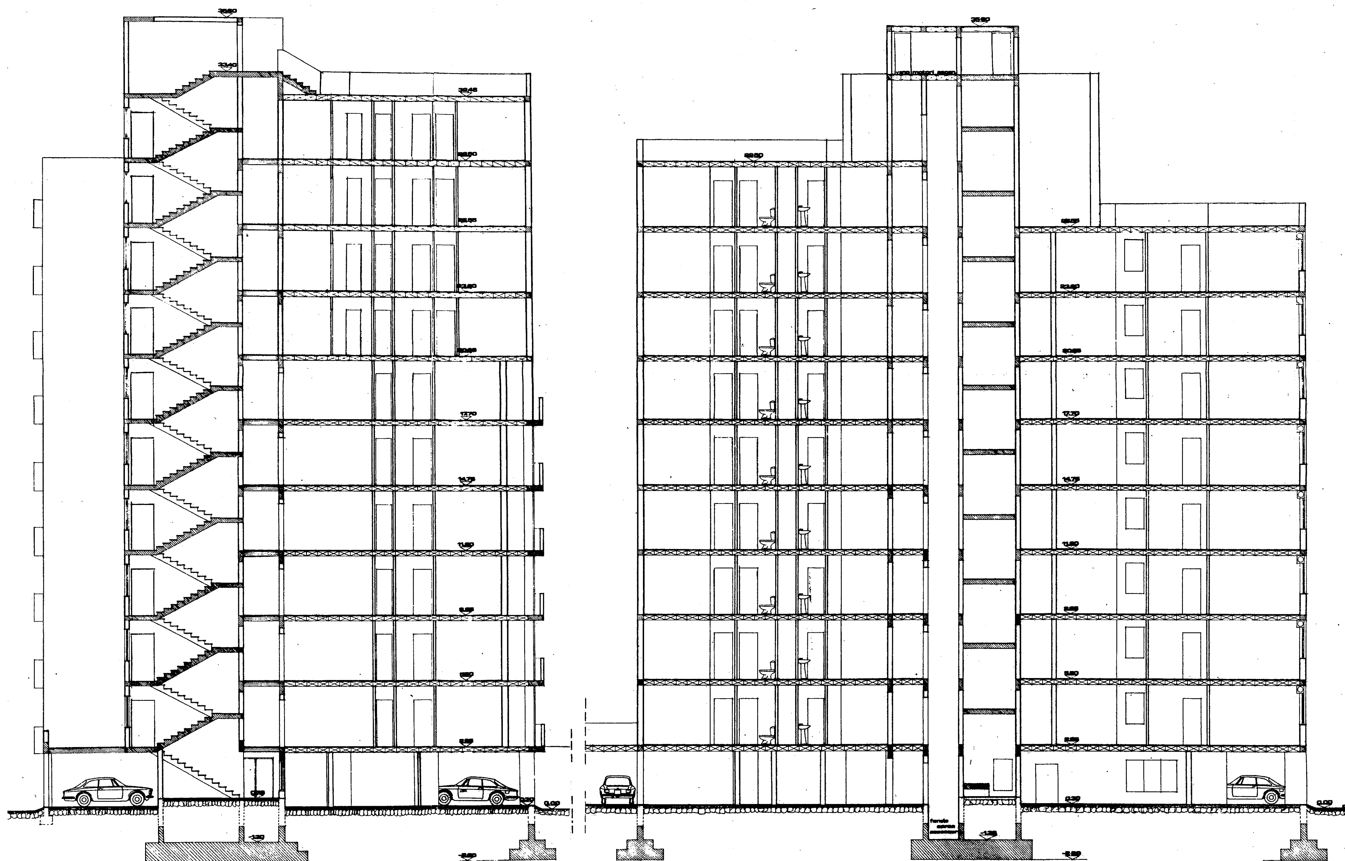
SEZIONE B-B
