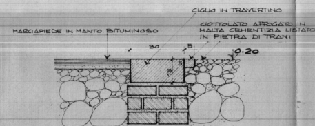
c PARTICOLARE ATTACCO MARCIAPIEDE CON BASAMENTO EDIFICIO rapp. 1:10
