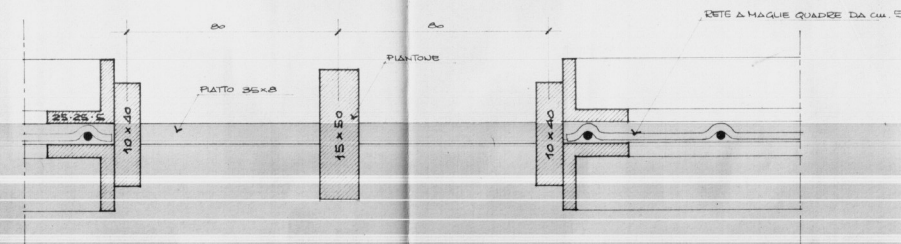
SEZIONE G rapp. 1:1
