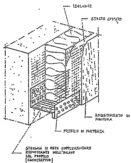
Profilo di base con gocciolatoio (o profilo di partenza)
