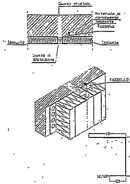
Profilo laterale utilizzato in prossimità di giunti di dilatazione
