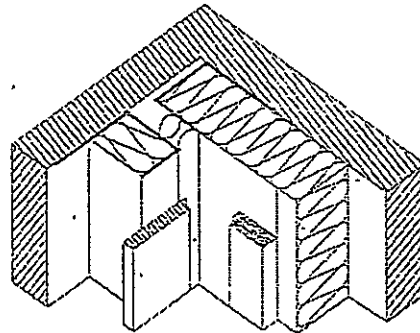
Profilo laterale utilizzato per angoli concavi
