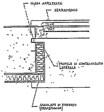
Profilo laterale utilizzato in prossimità di un vano finestra
