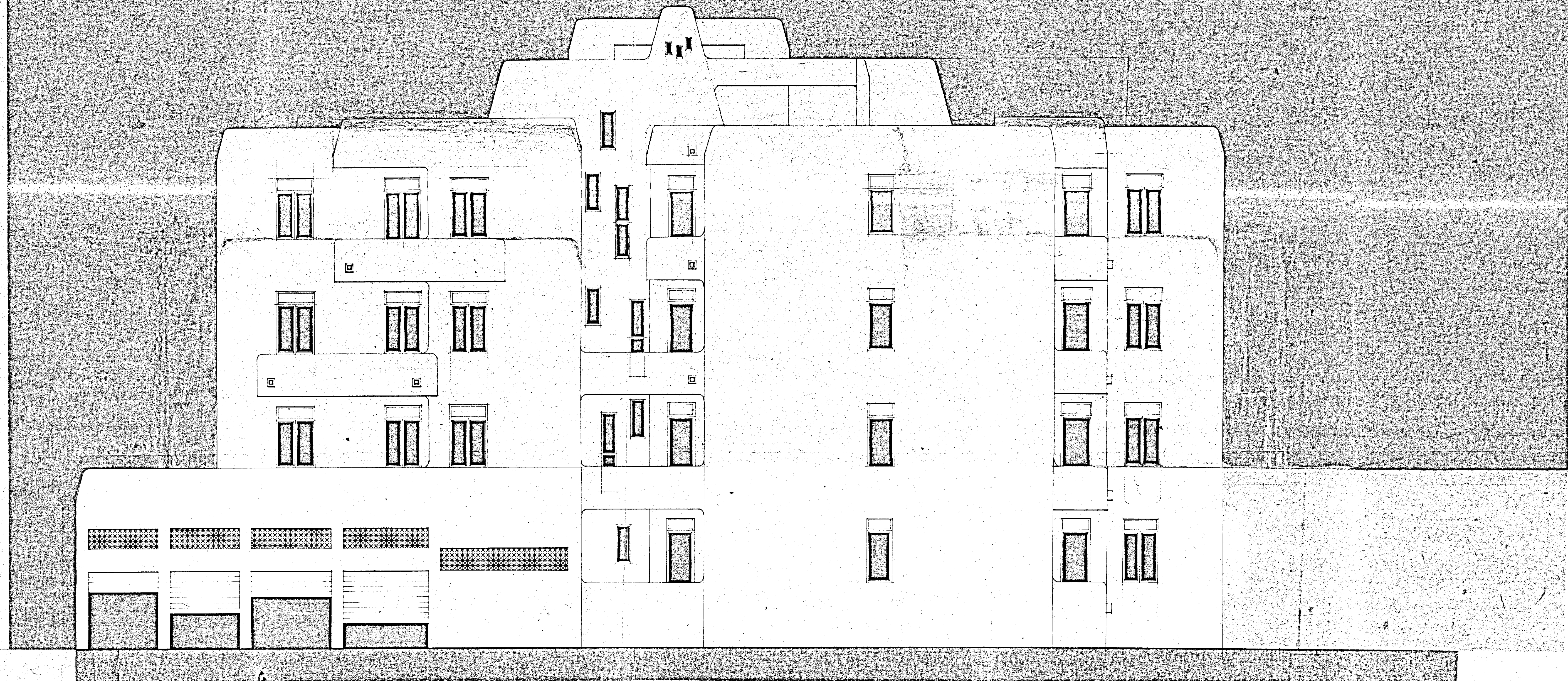
PROSPETTO - C-
