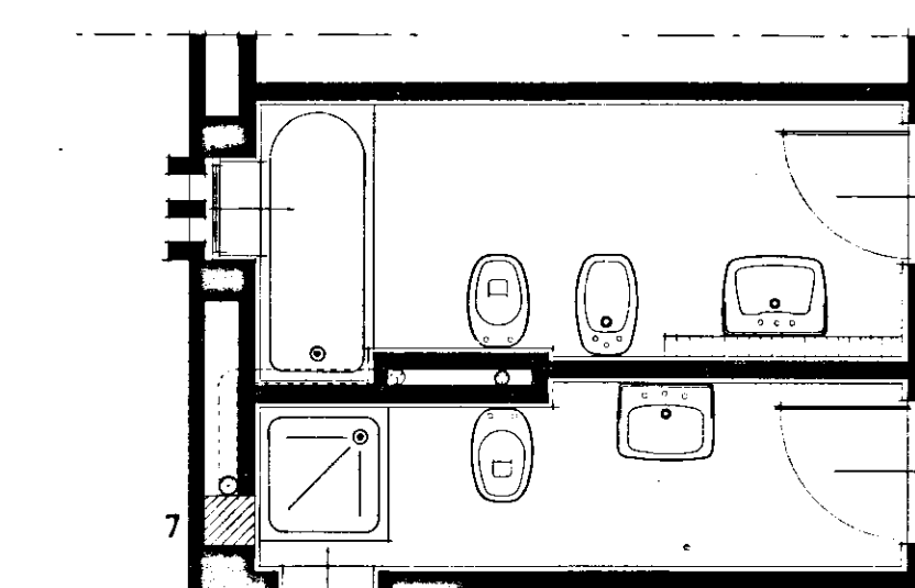
Appartam. C Particolare bagni al 1° piano: vasi con scarico a parete.
