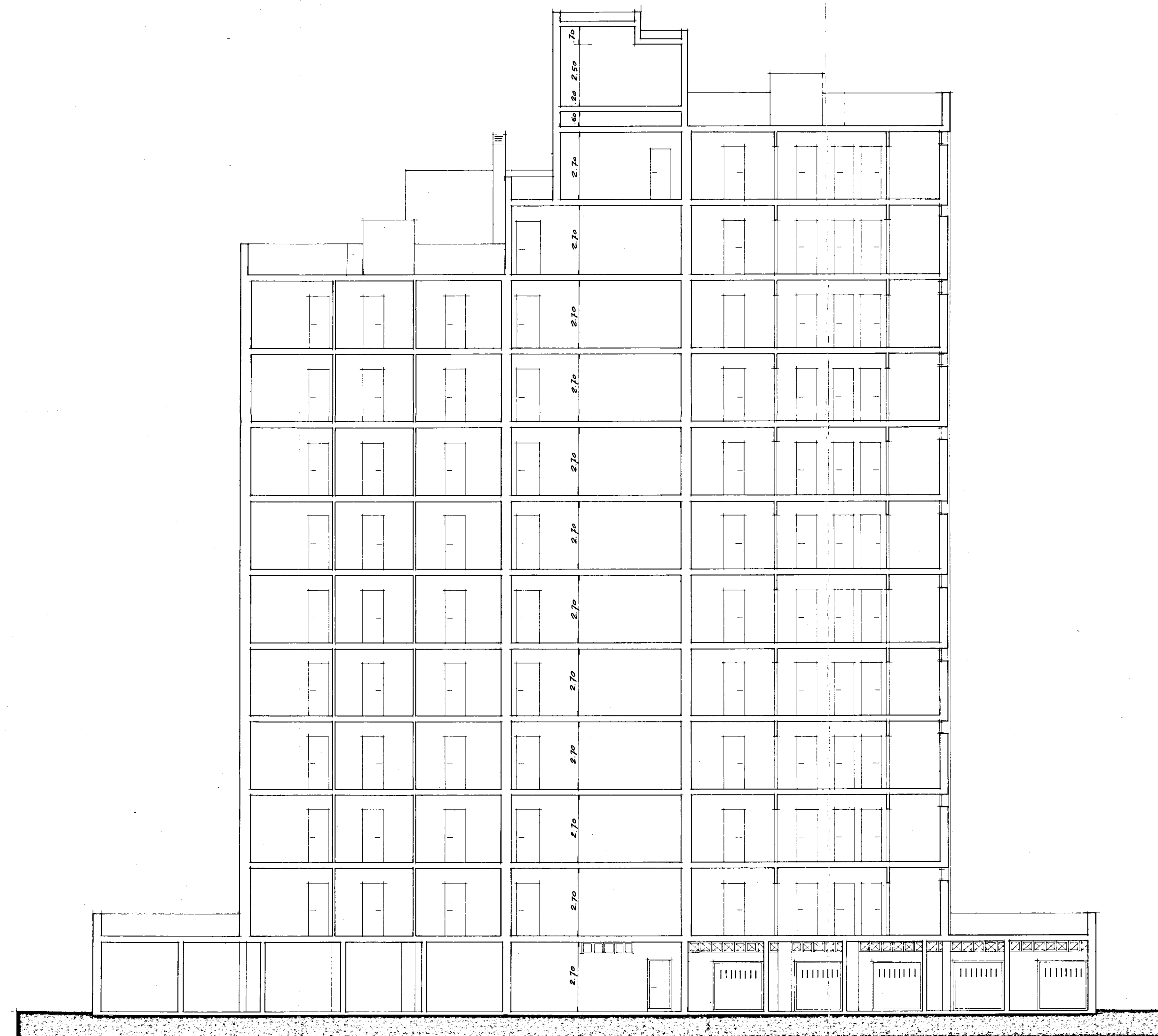
SEZIONE X - X
