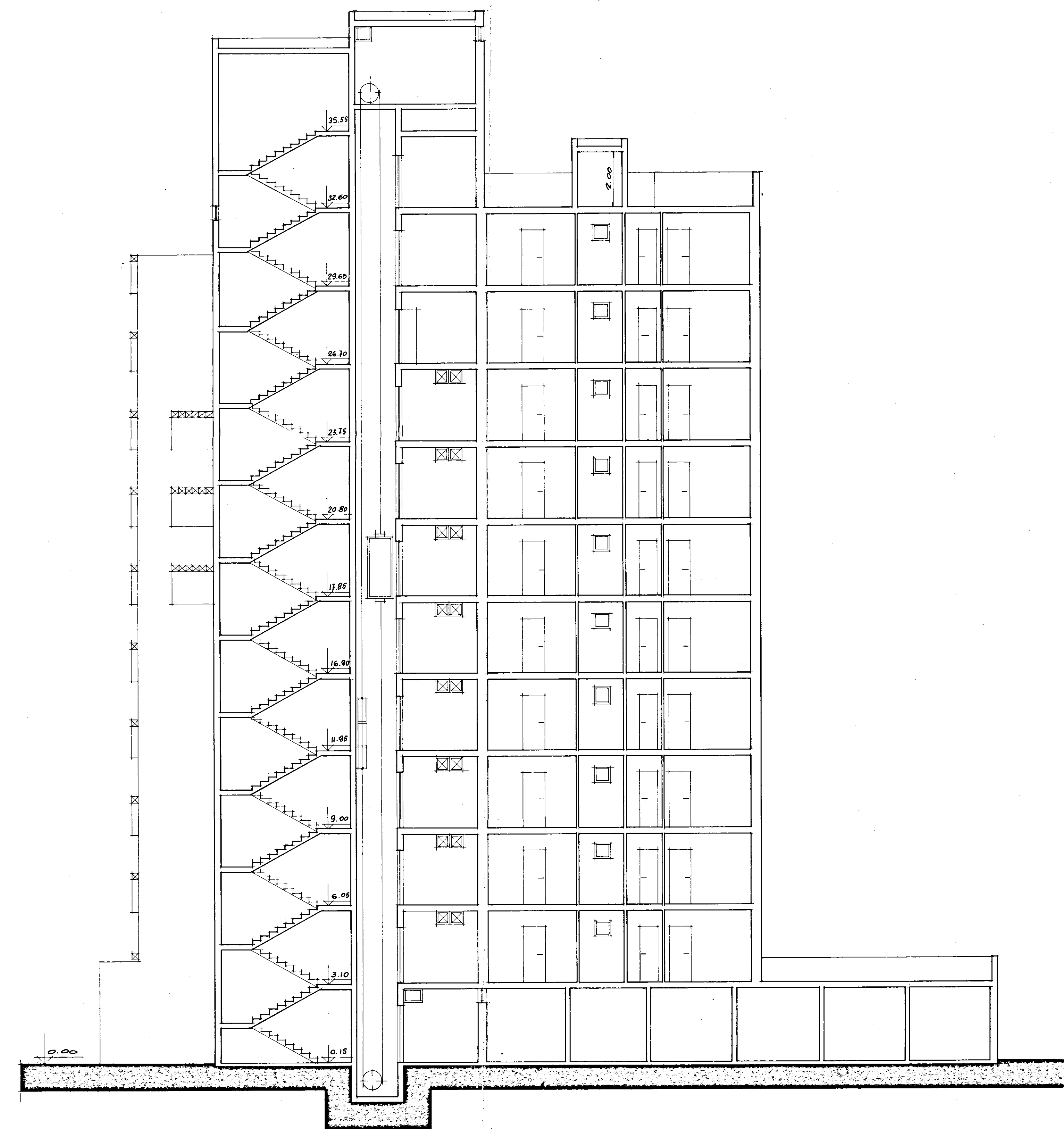
SEZIONE Y - Y
