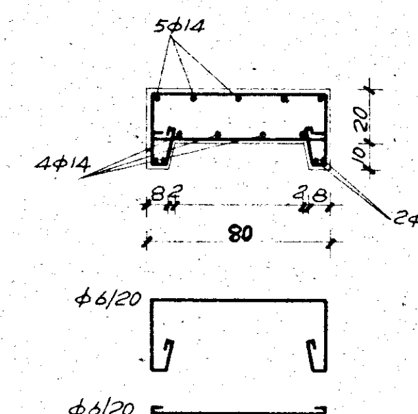
SEZIONE TRAVE DI CORONAMENTO PORTICO RAPP. 1:20
