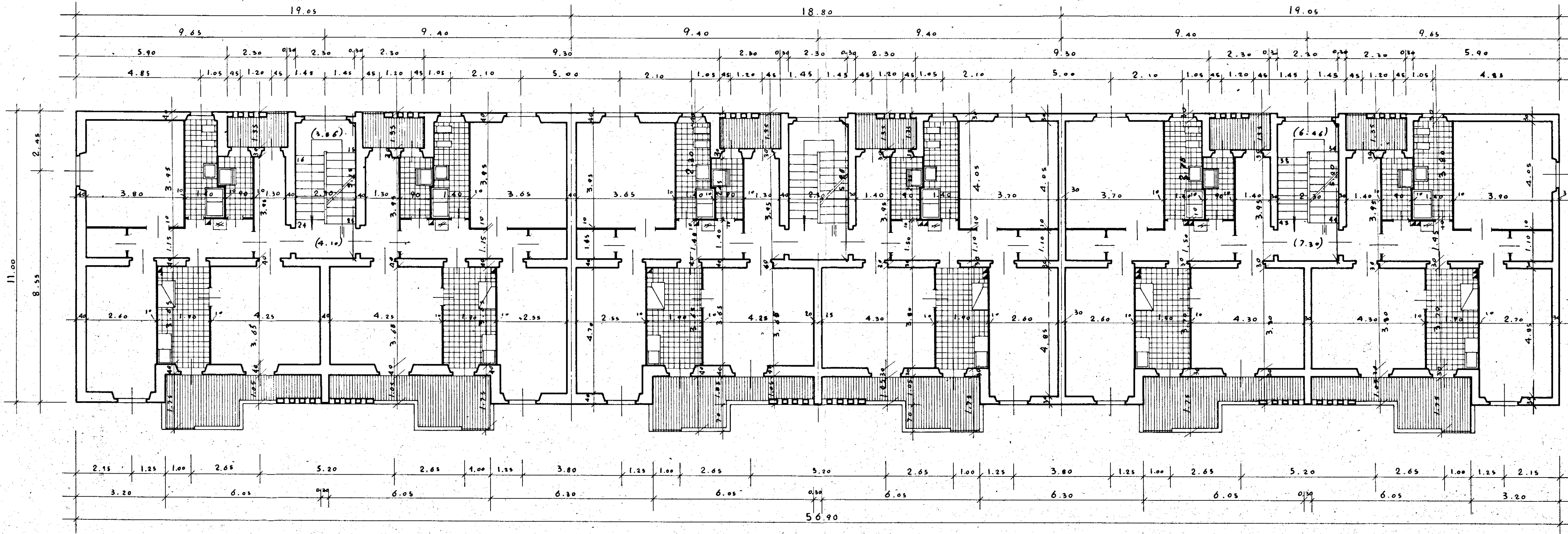
DIS. N° 122 PIANTE PIANI 1° E 2° RAPP. 1:100
