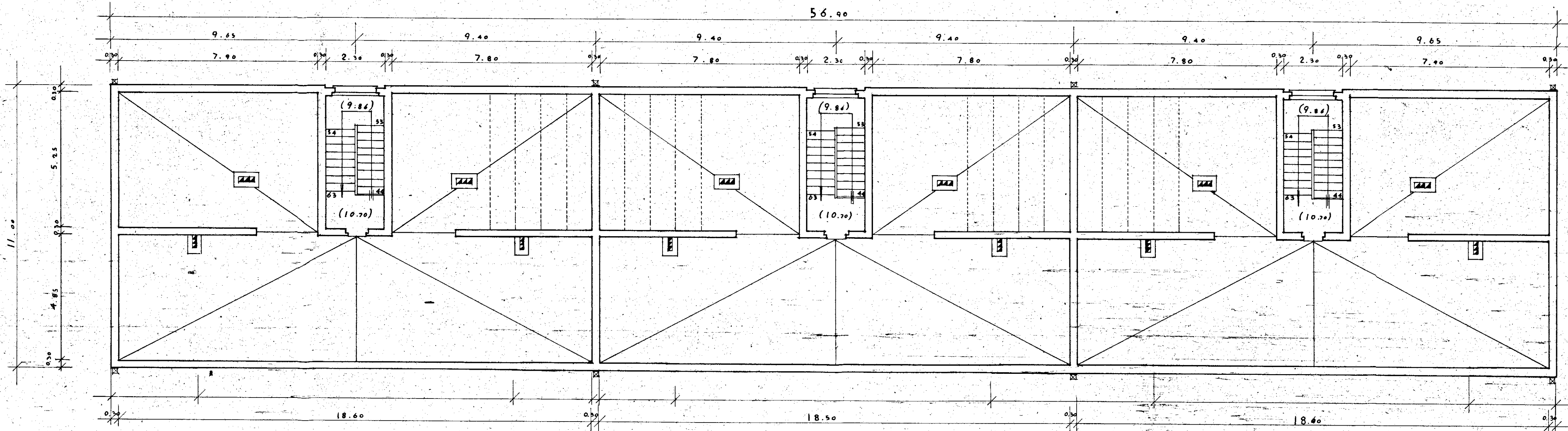
DIS. N° 123 PIANTA PIANO COPERTURA RAPP. 1:100
