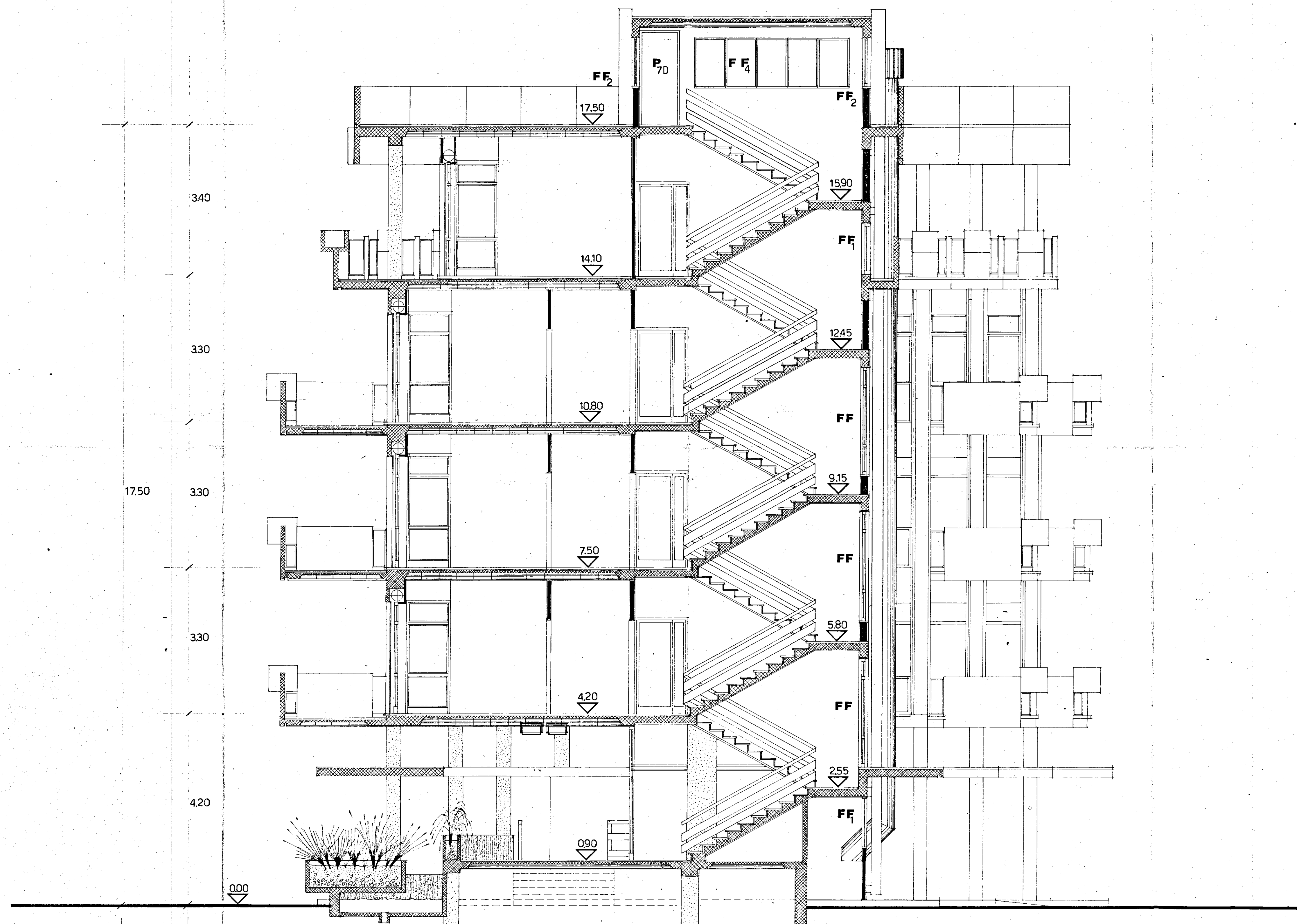
SEZIONE A-B RAPP. 1/50
