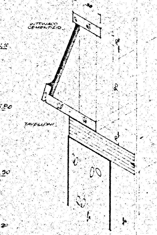
NODO "A" VISTA ASSONOMETRICA
