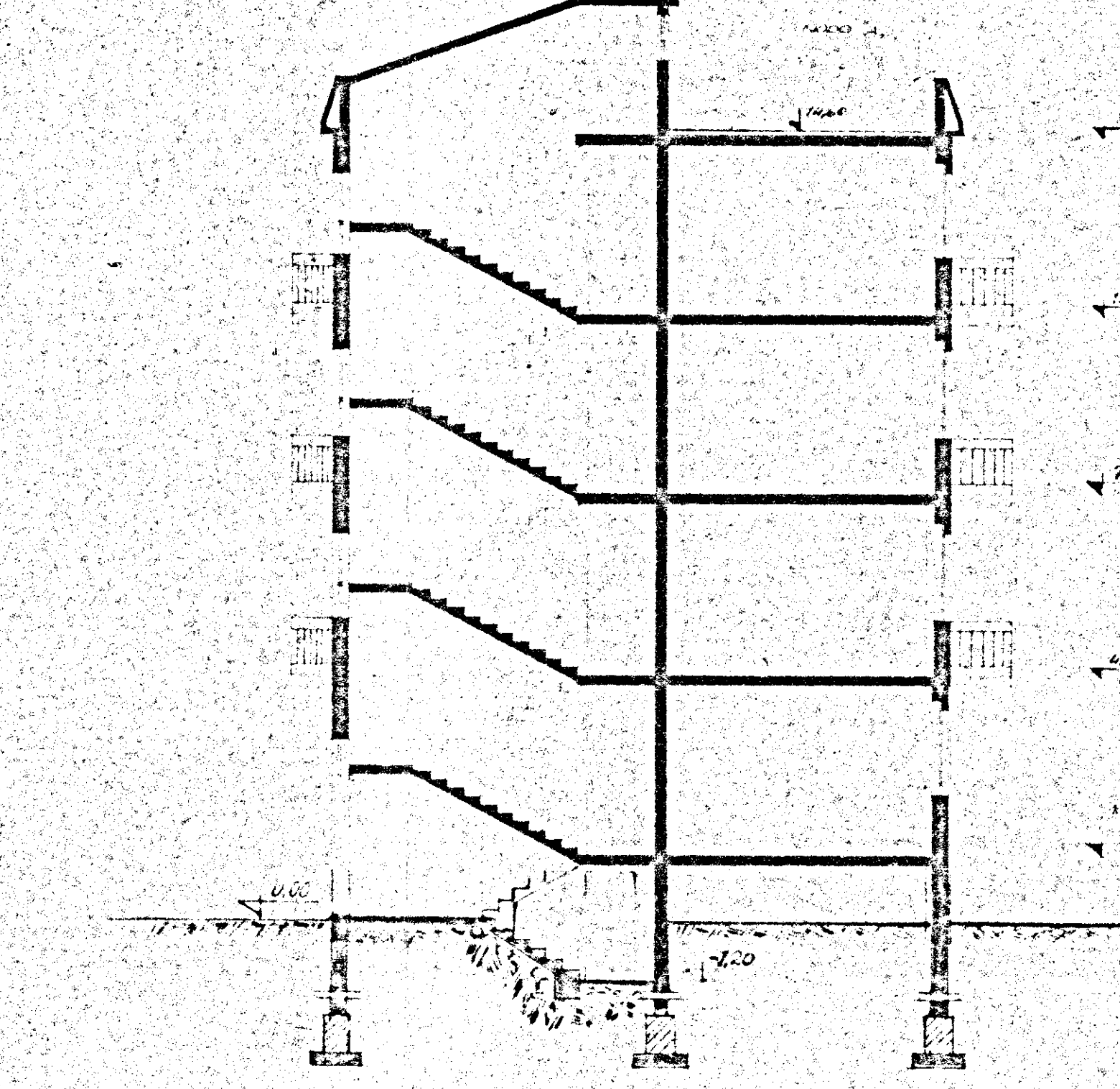
SEZIONE A-X
