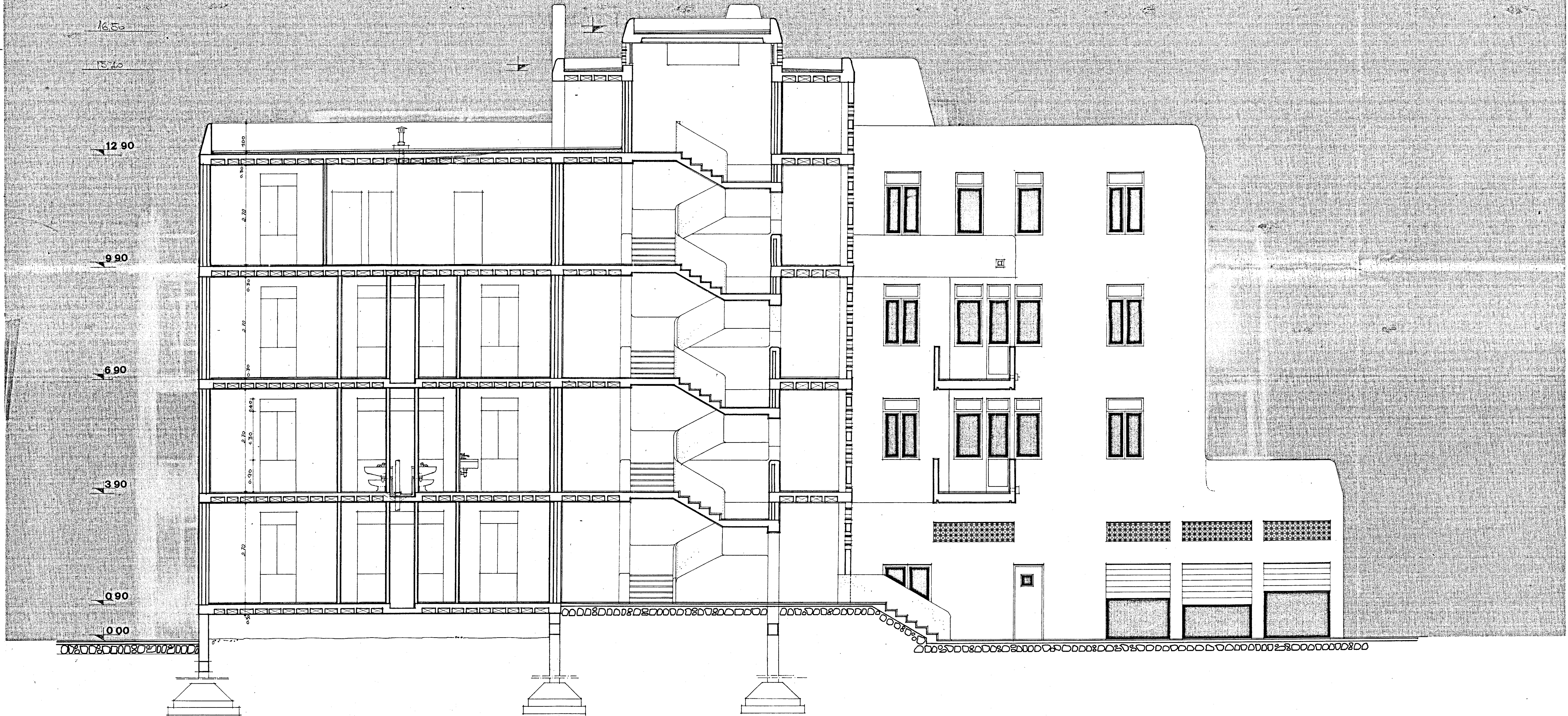
SEZIONE A-A'
