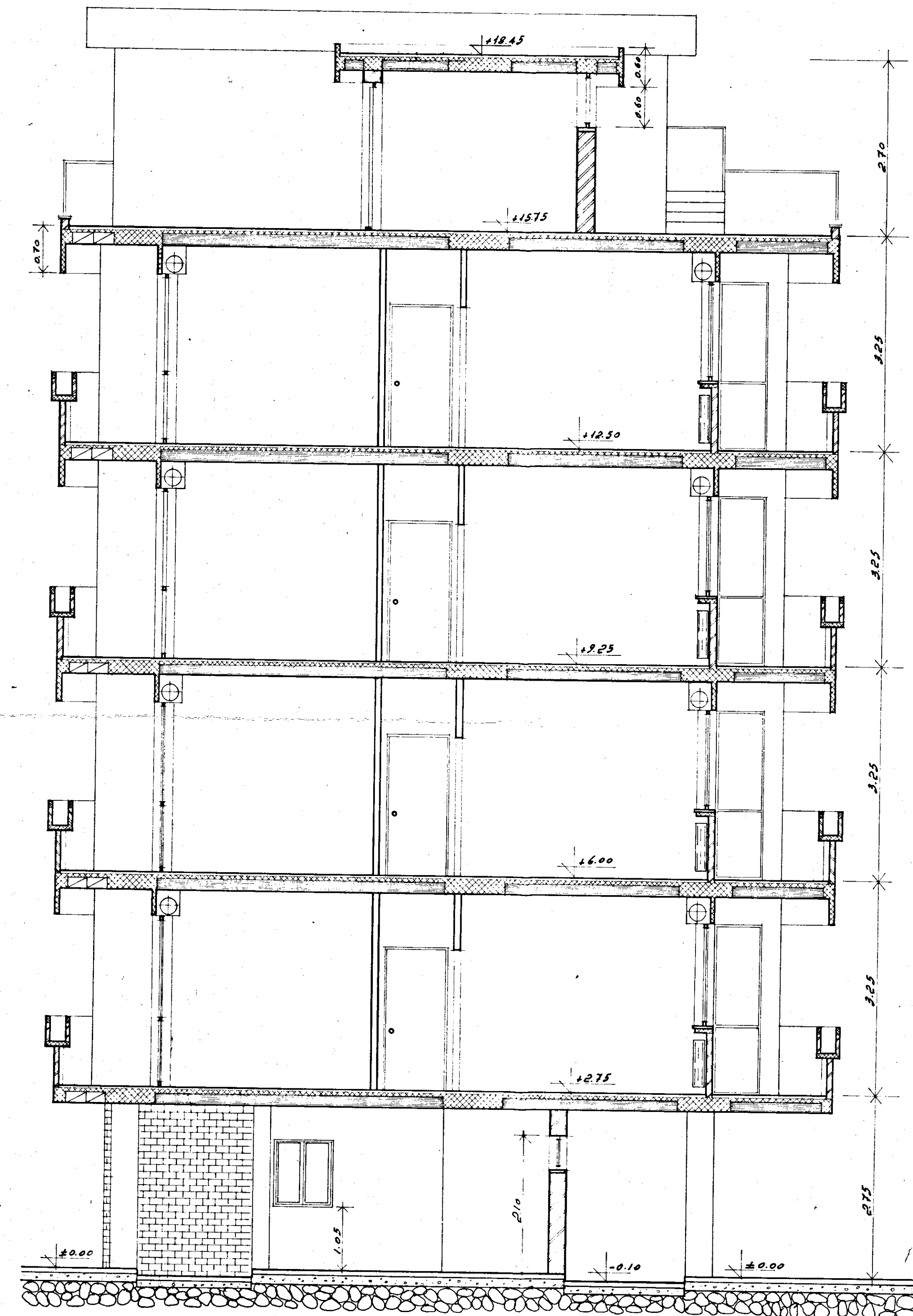
SEZ. C-C
