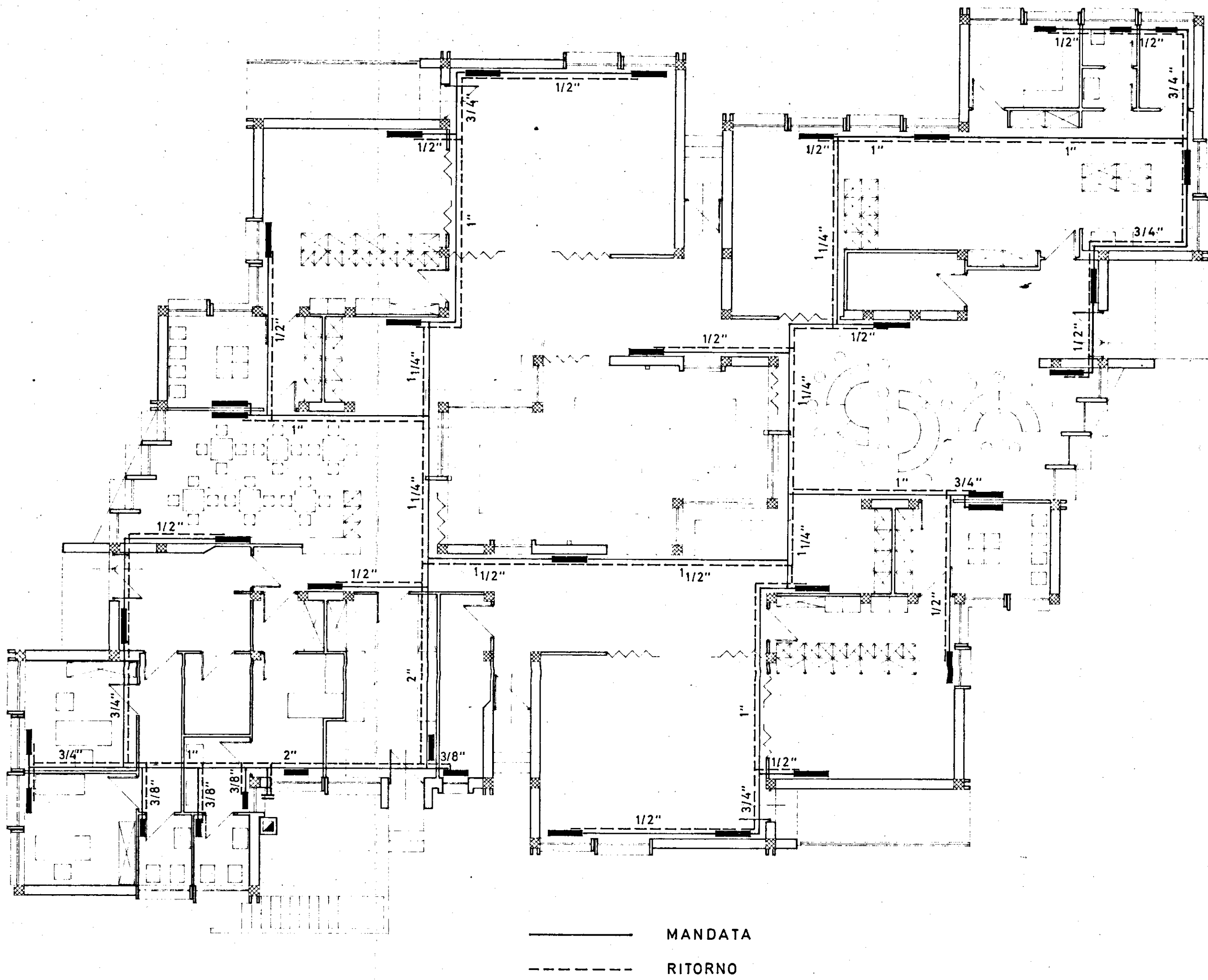
IMPIANTO TERMICO
