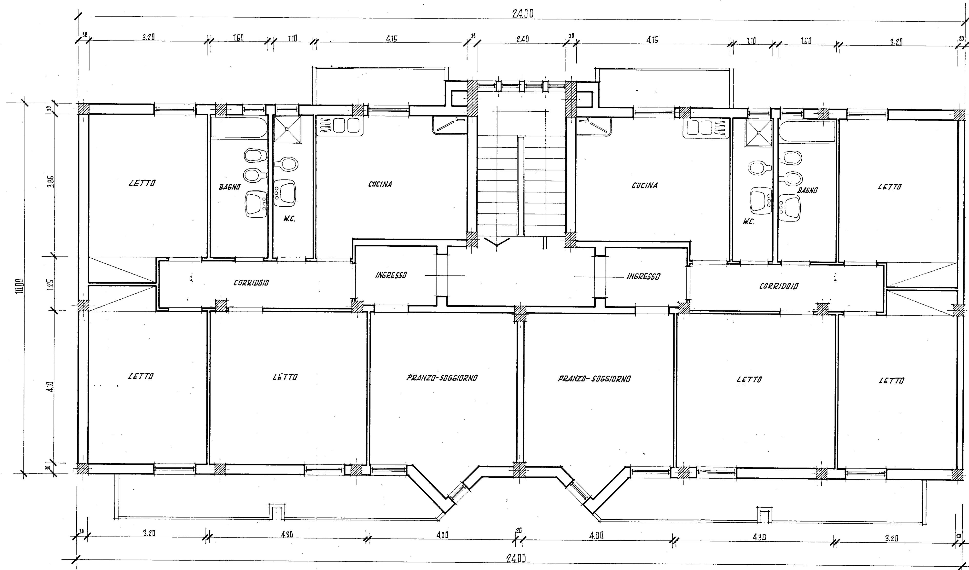
PIANTA 1° E 2° PIANO SCALA 1:50
