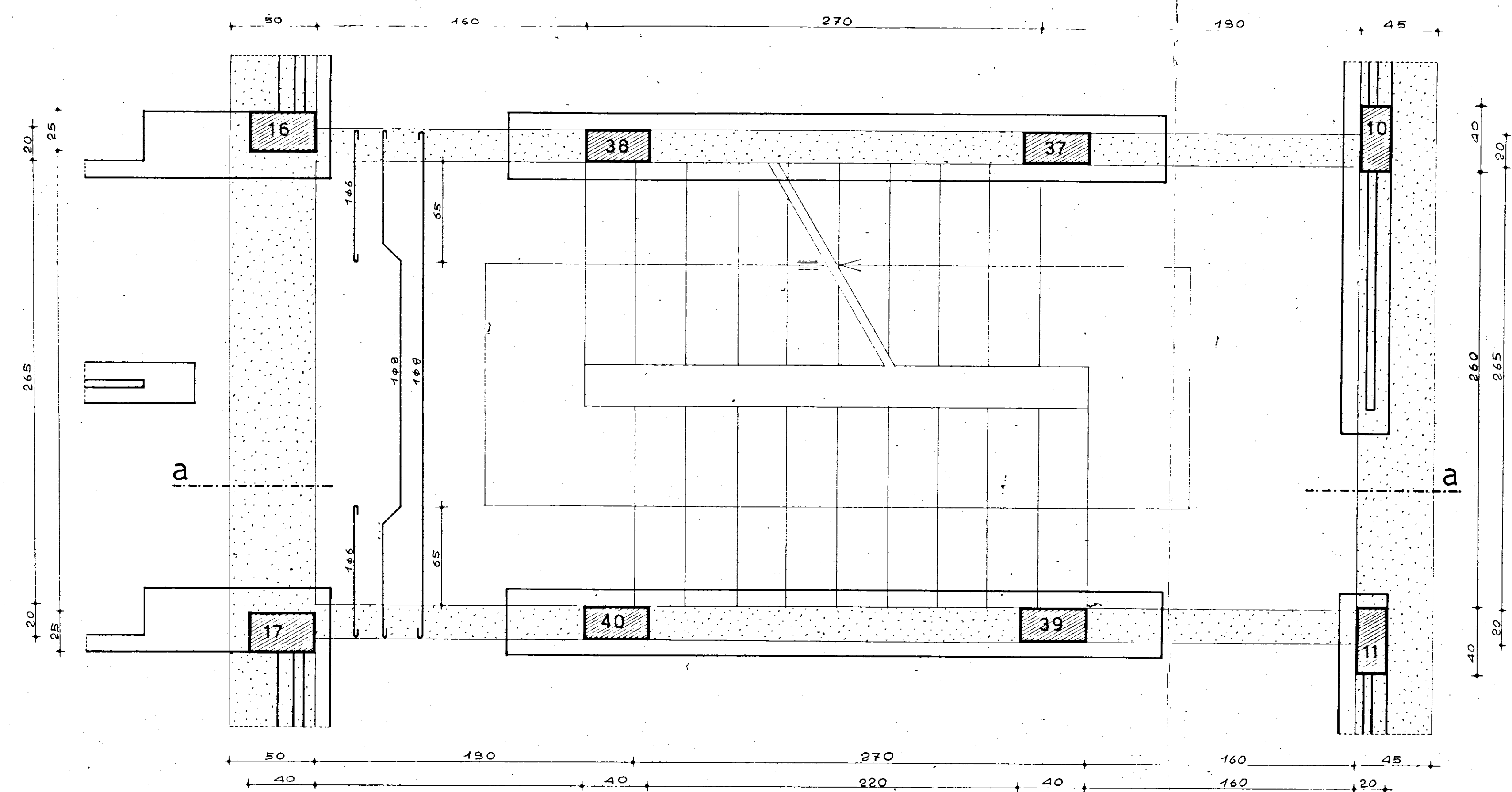
piano tipo
