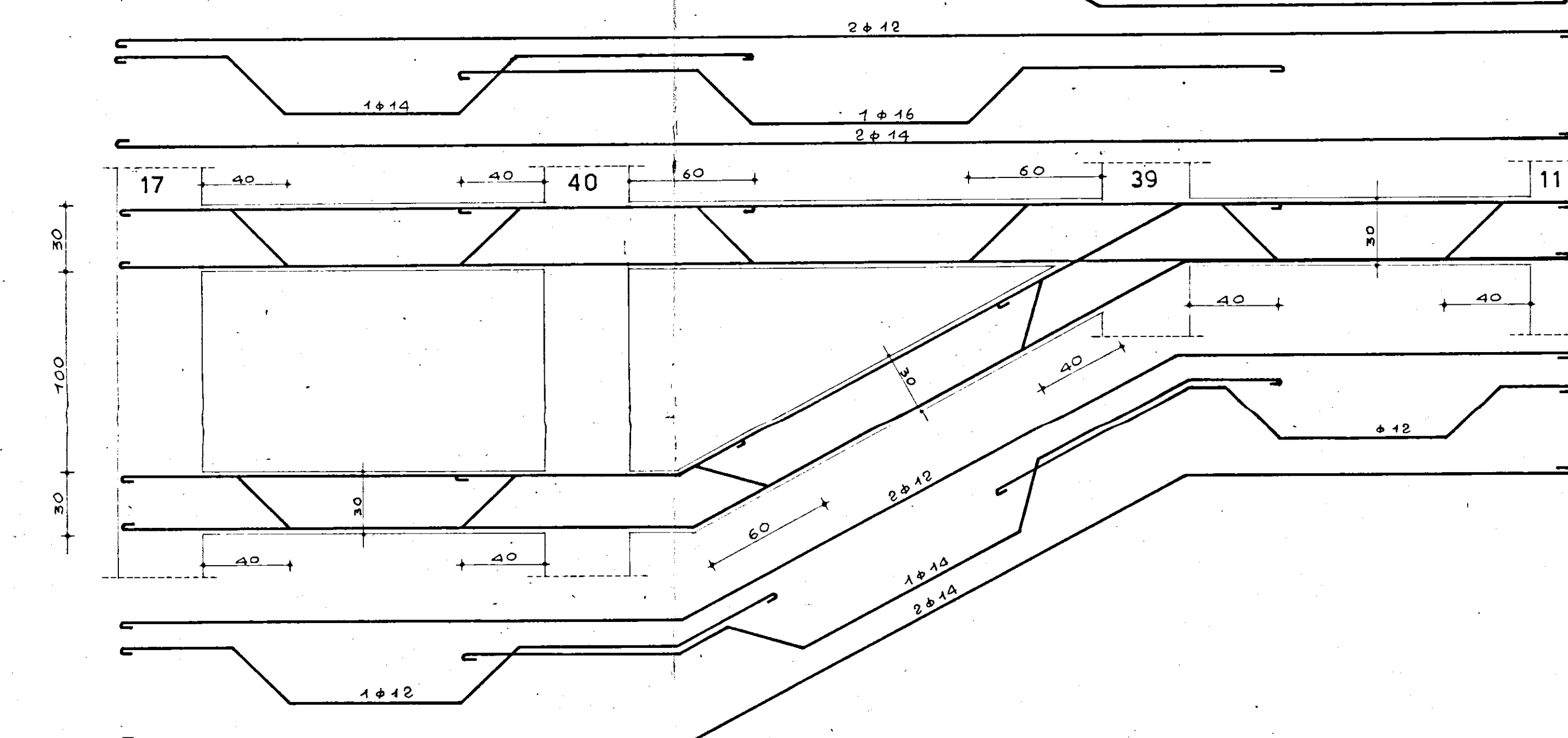
sez. b-b
