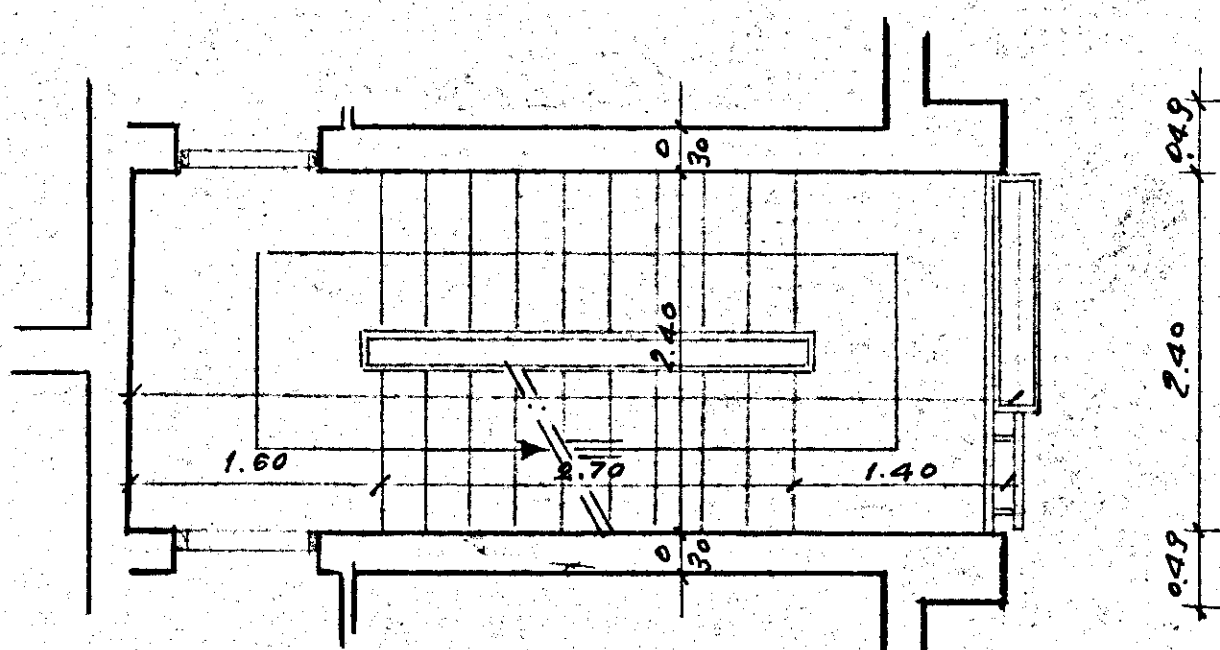
FABBRICATO 7/2 - SCALA PIANO TIPO Rapp. 1:50
