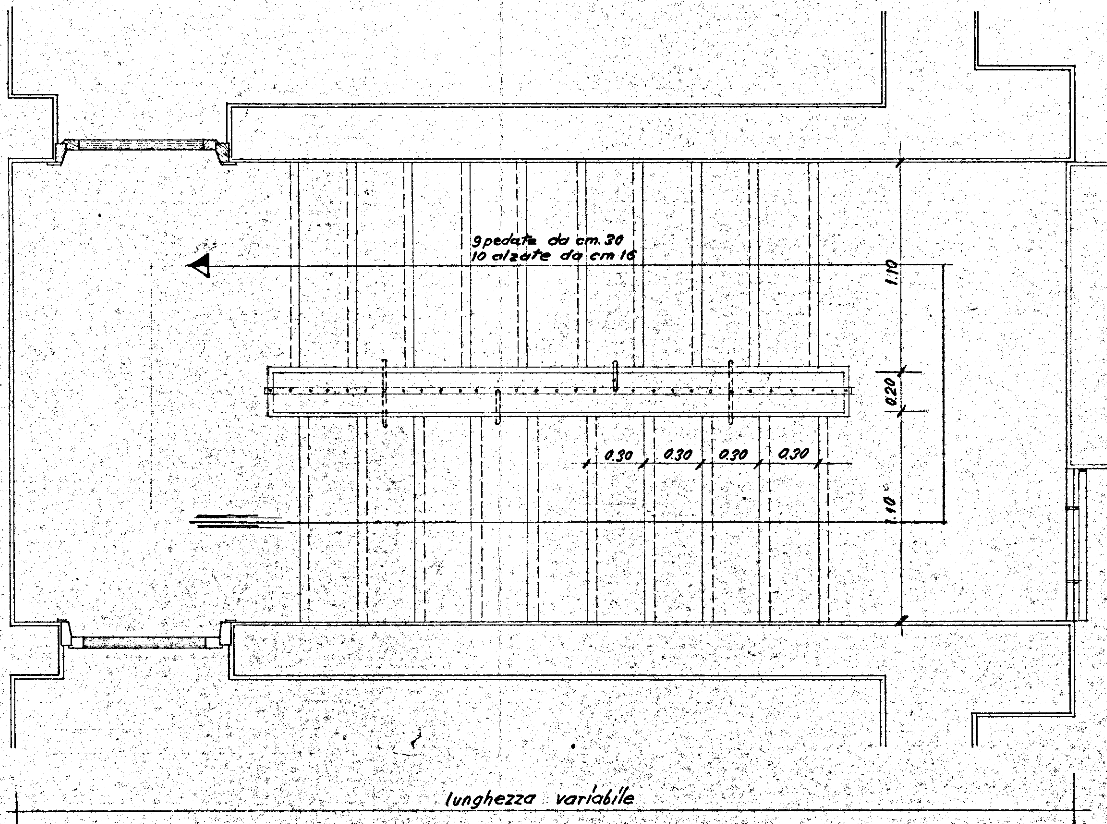
DIANTA Rapp. 1:20
