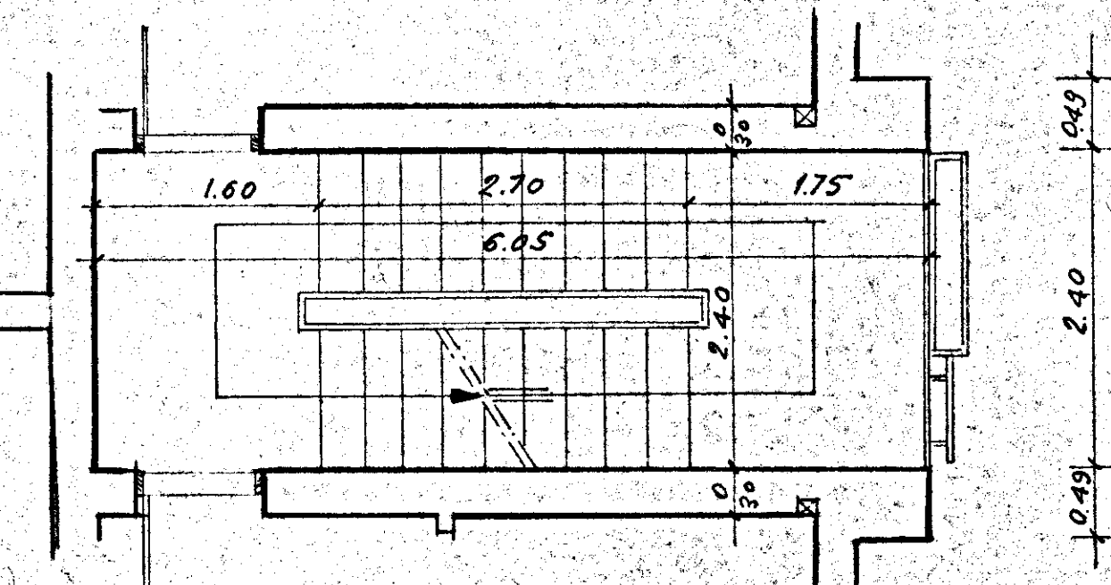
FABBRICATO 7/3 - SCALA PIANO TIPO Rapp. 1:50
