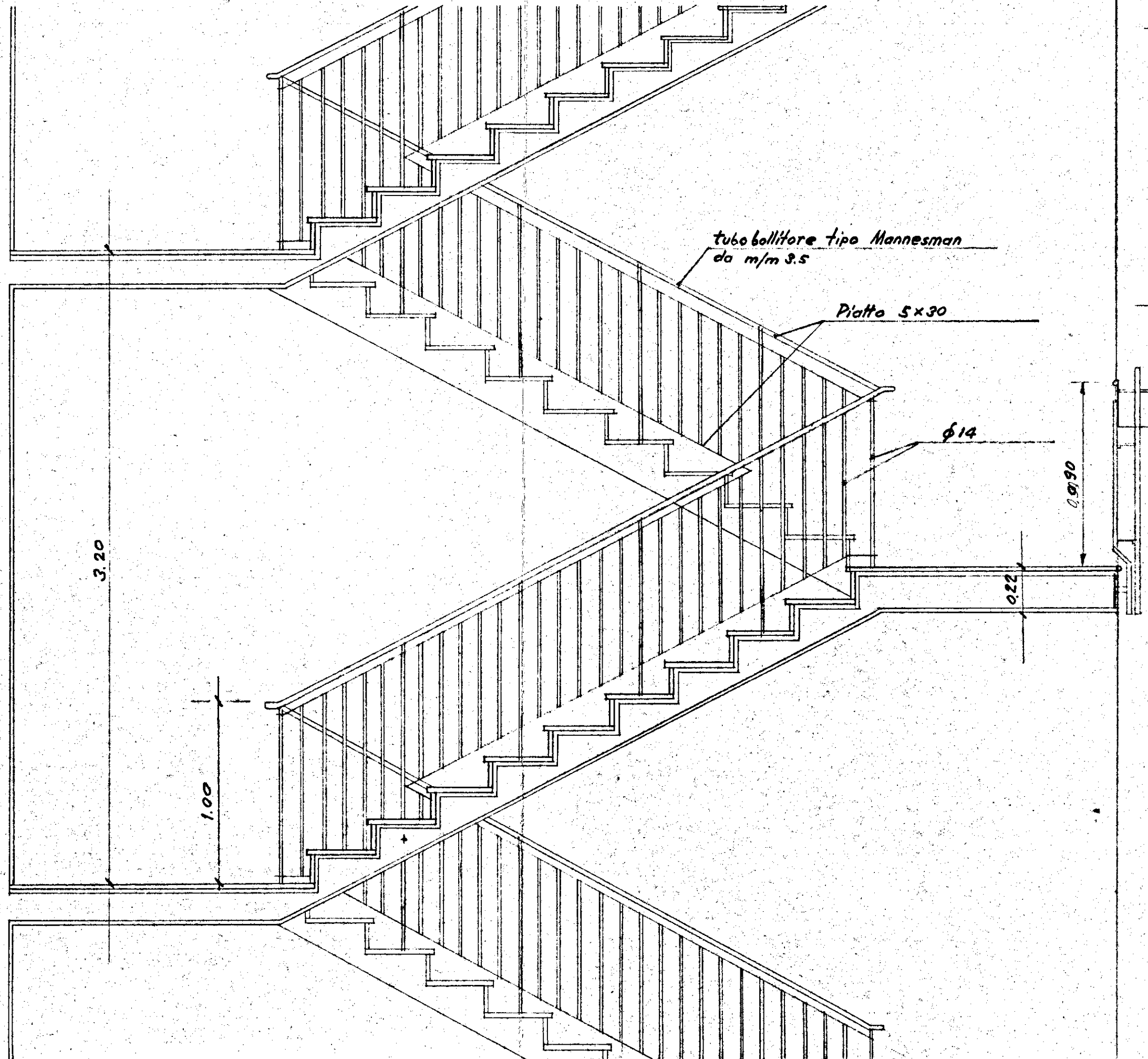
ALZATA Rapp. 1:20
