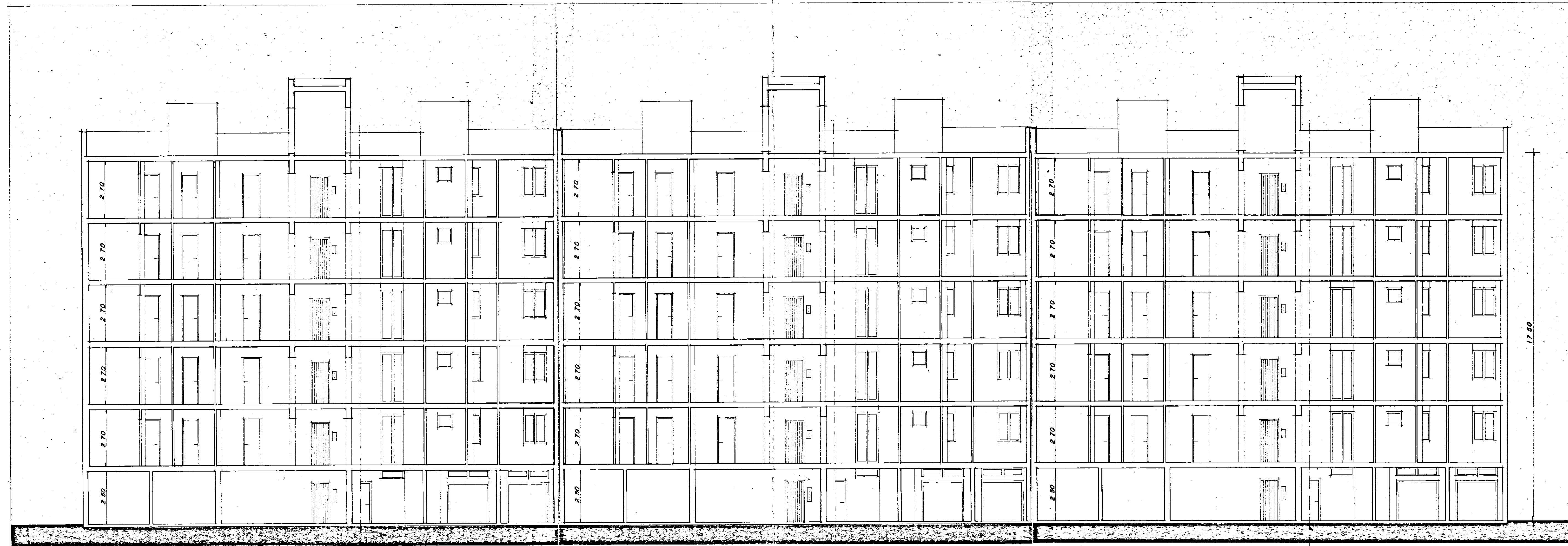
SEZIONE X-X
