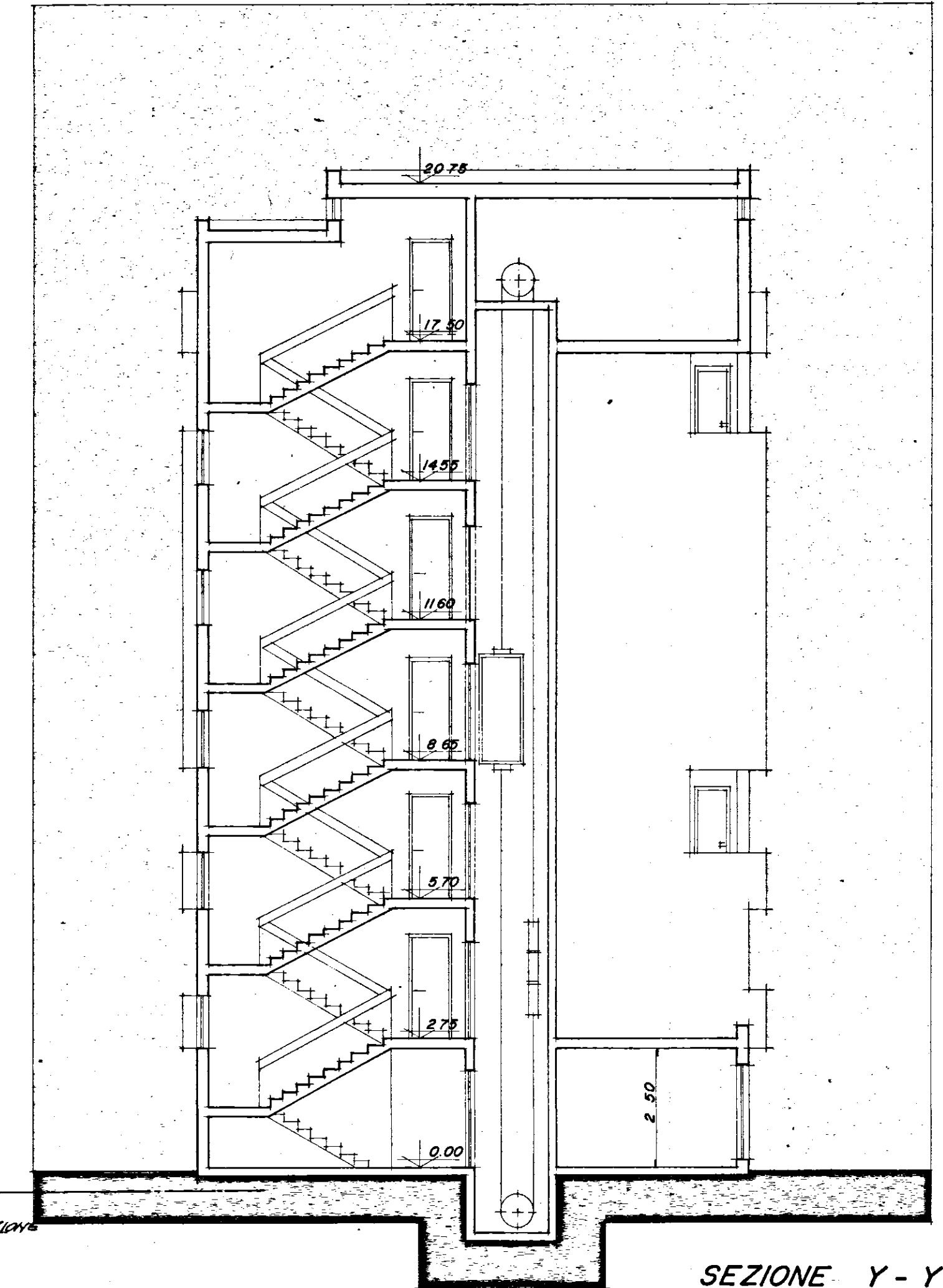
SEZIONE Y-Y
