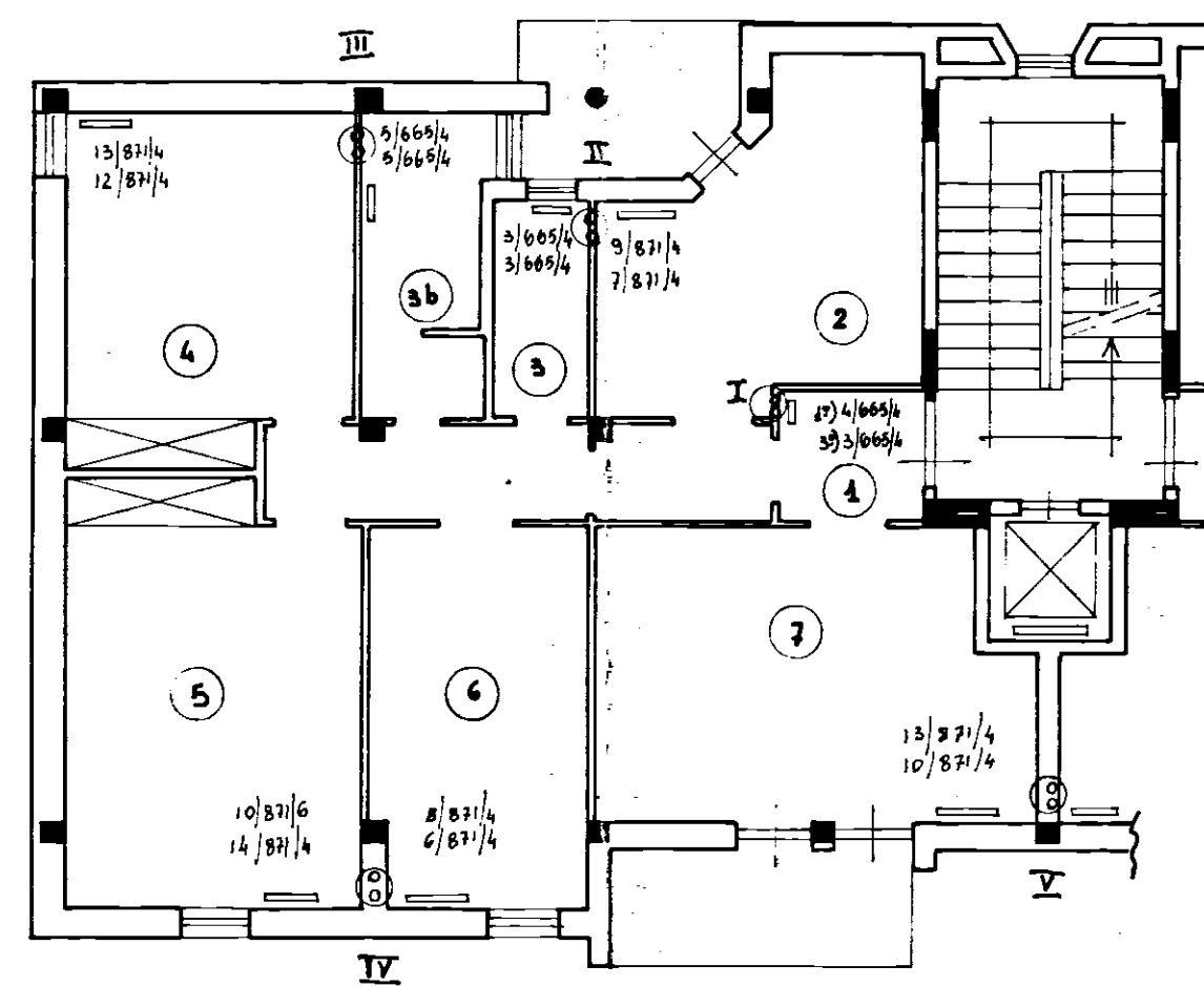
VARIANTE AL 1° e 3° PIANO
