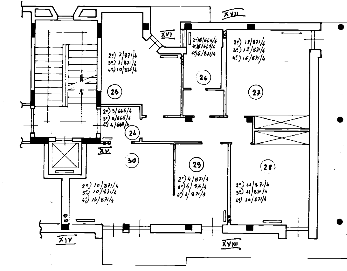
VARIANTE AL 2°-3°-4°-PIANO
