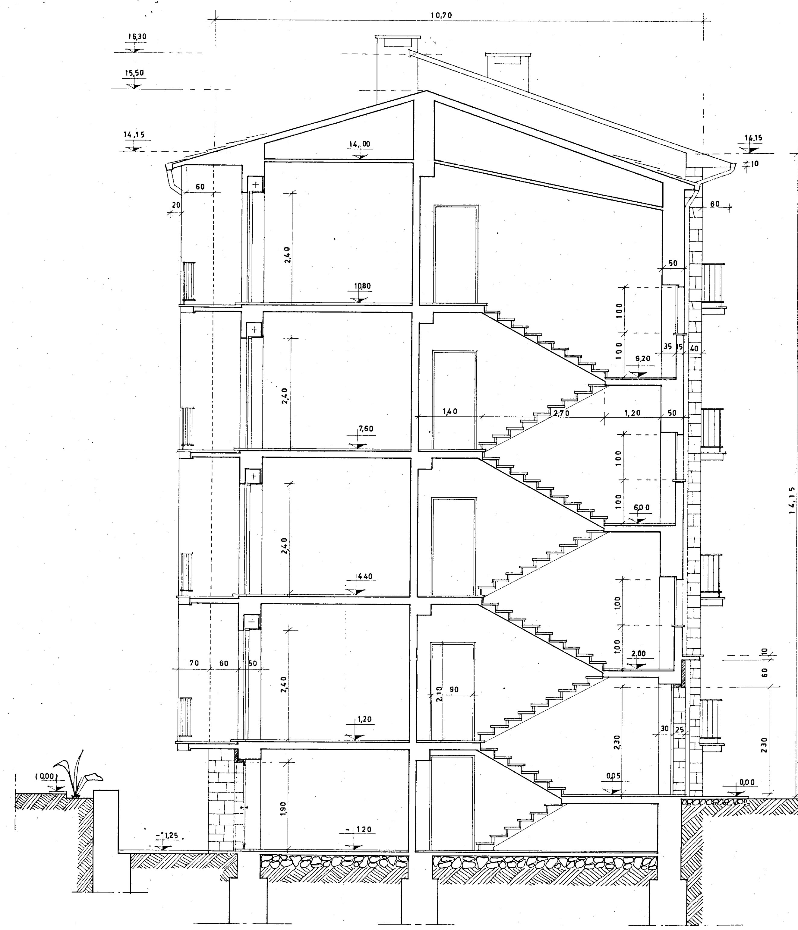
SEZIONE A-B RAPP. 1:50
