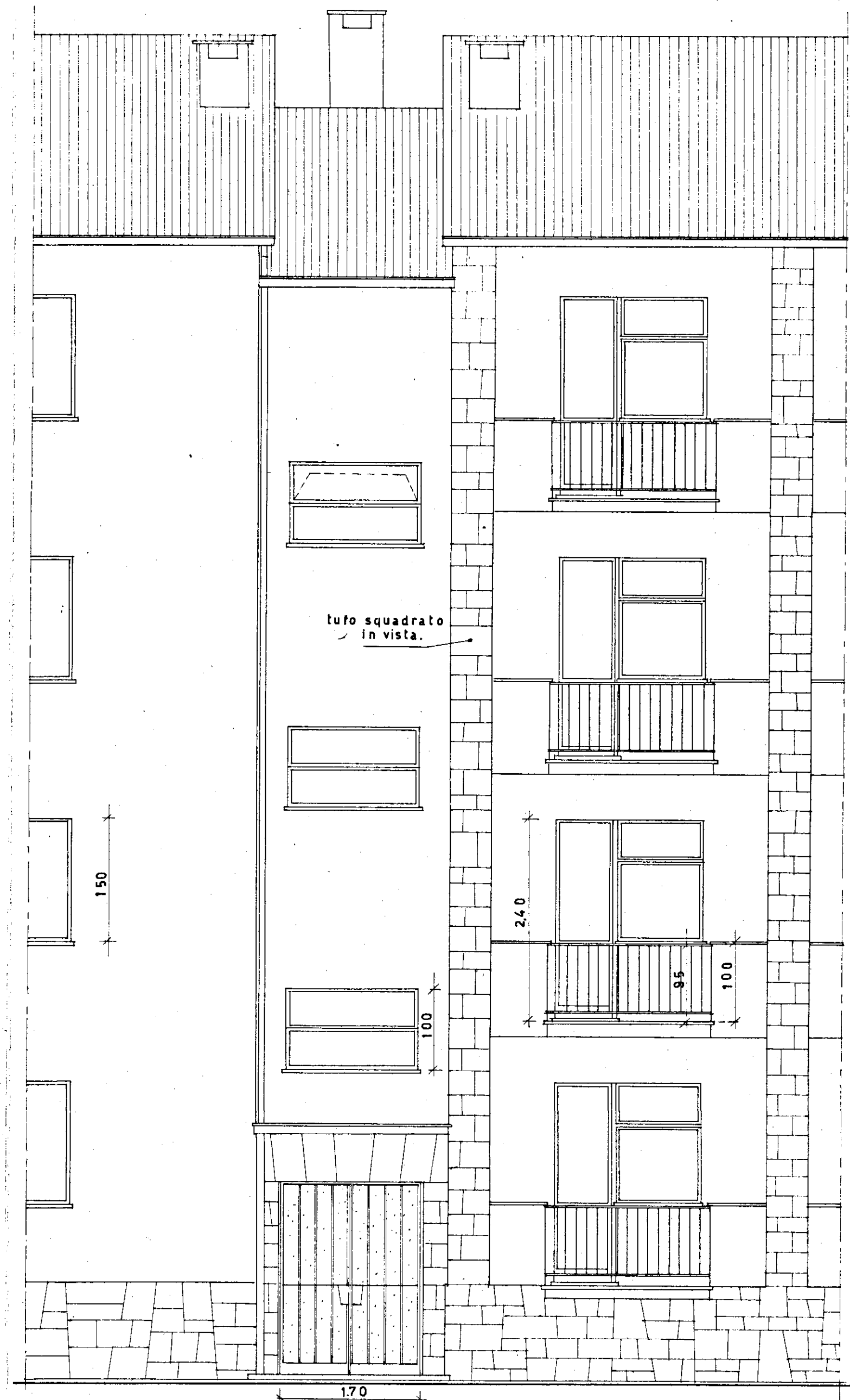
PARTICOLARE PROSPETTO LATO INGRESSO (Lato scala) RAPP. 1:50
