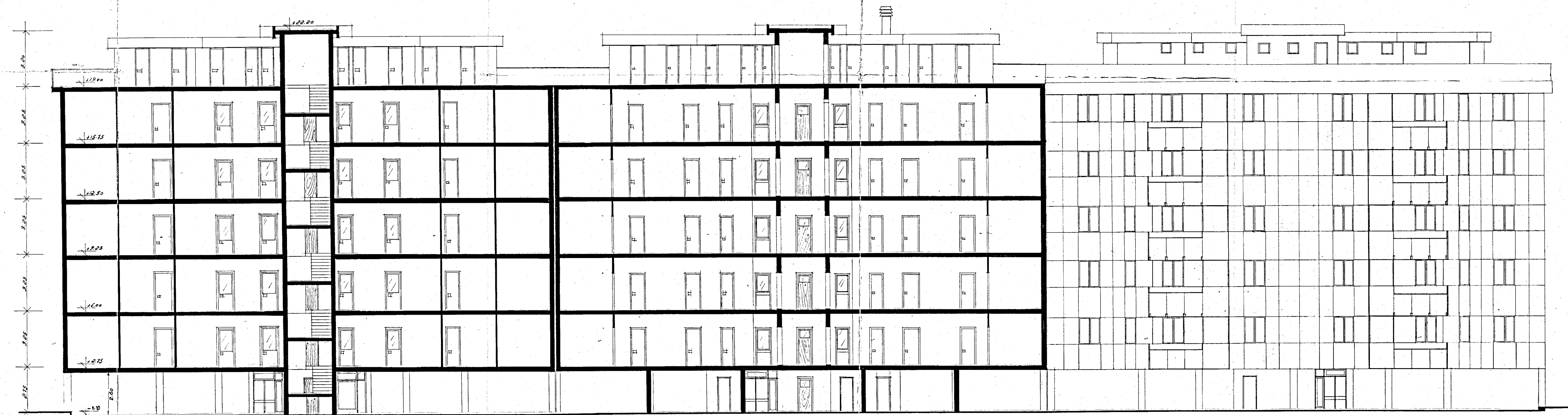
SEZ. X-X
