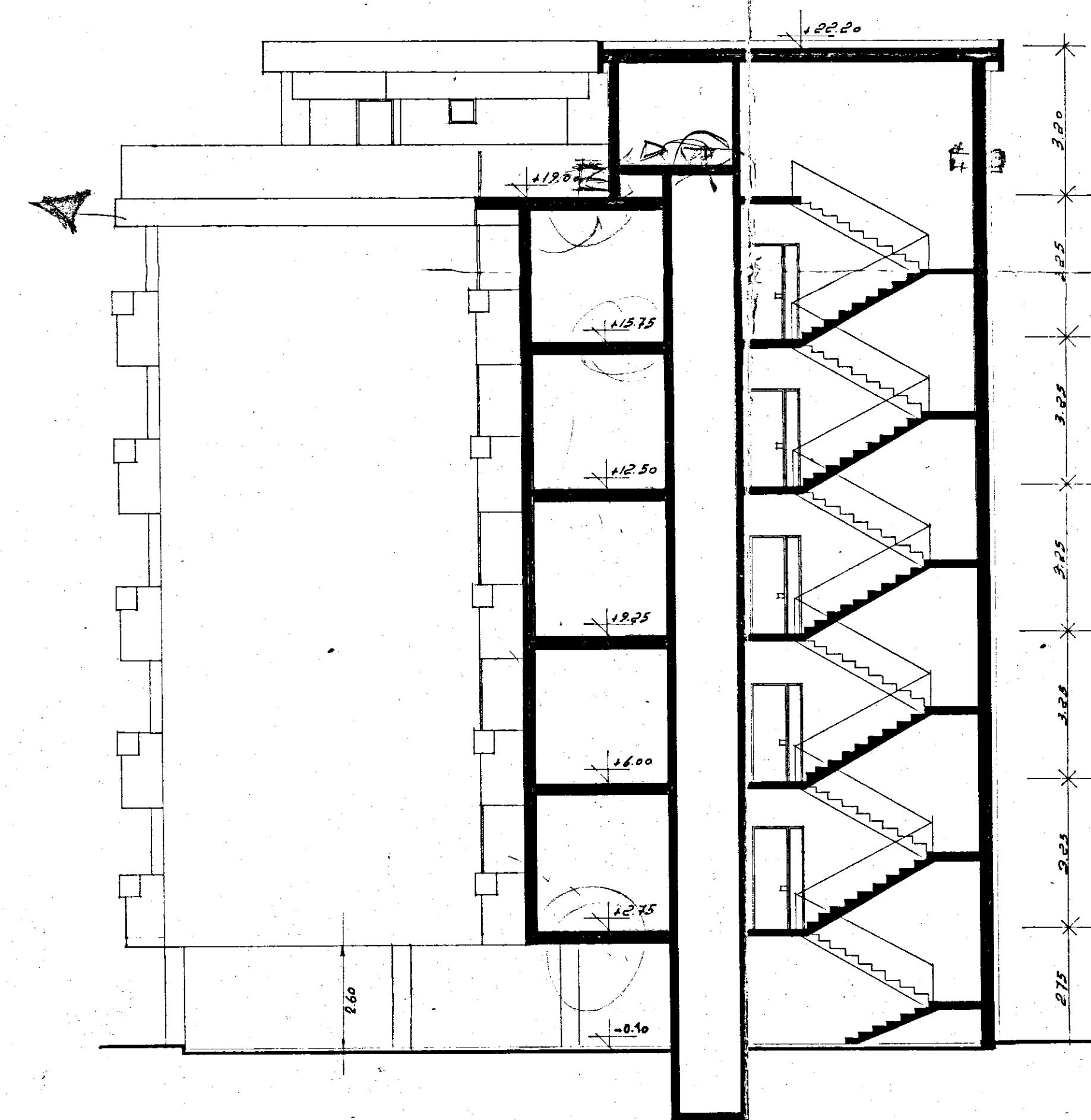
SEZ. F-F
