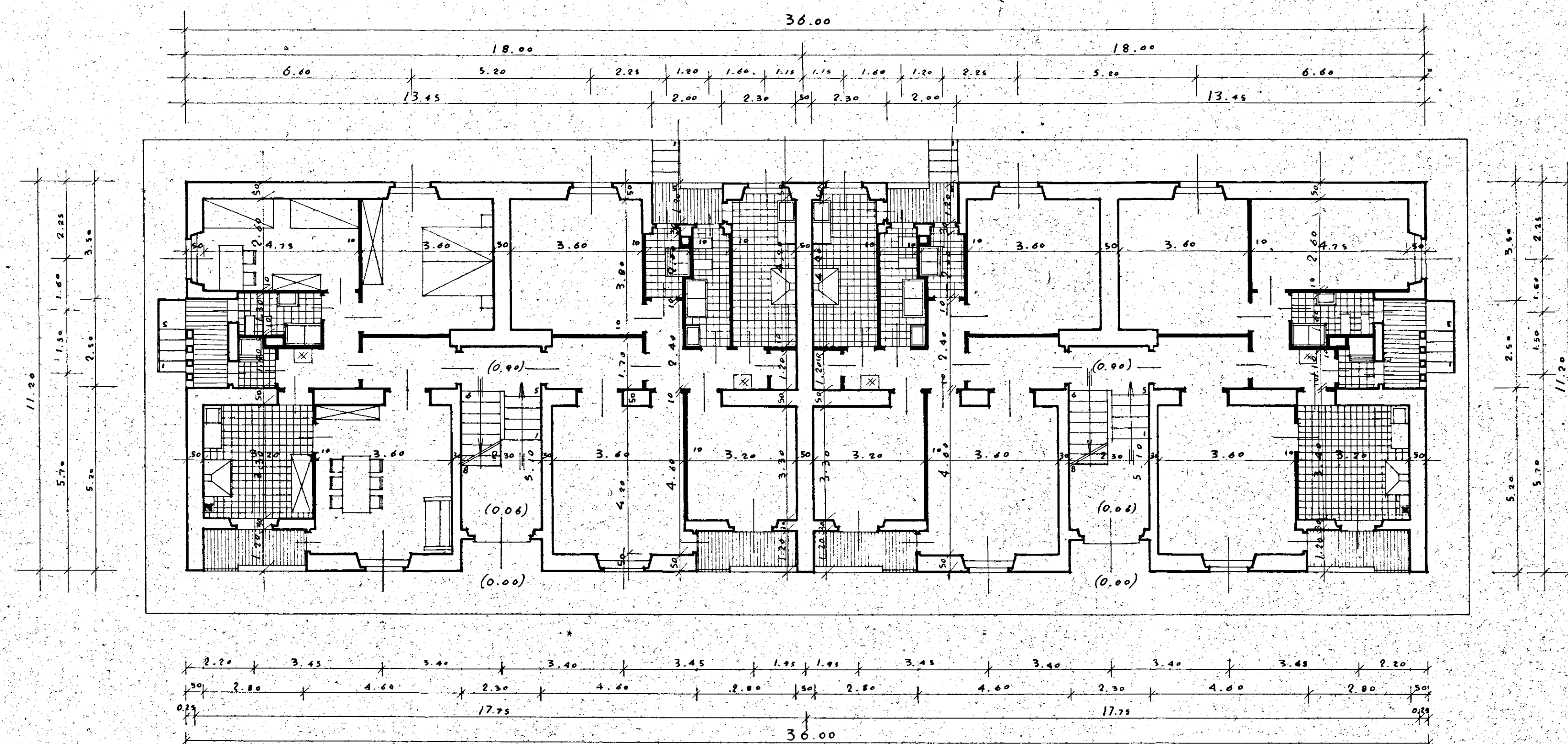
DIS. 68 PIANTE PIANO RIALZATO RAPP. 1:100
