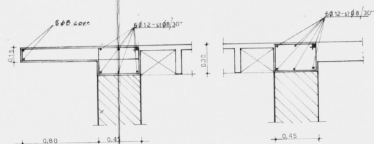
Sezione A-B
