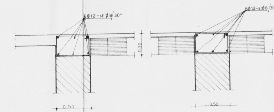
Sezione C-D
