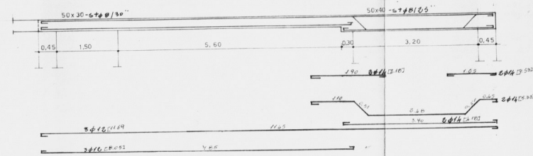
Armatura trave e cordolo sul muro di spina
