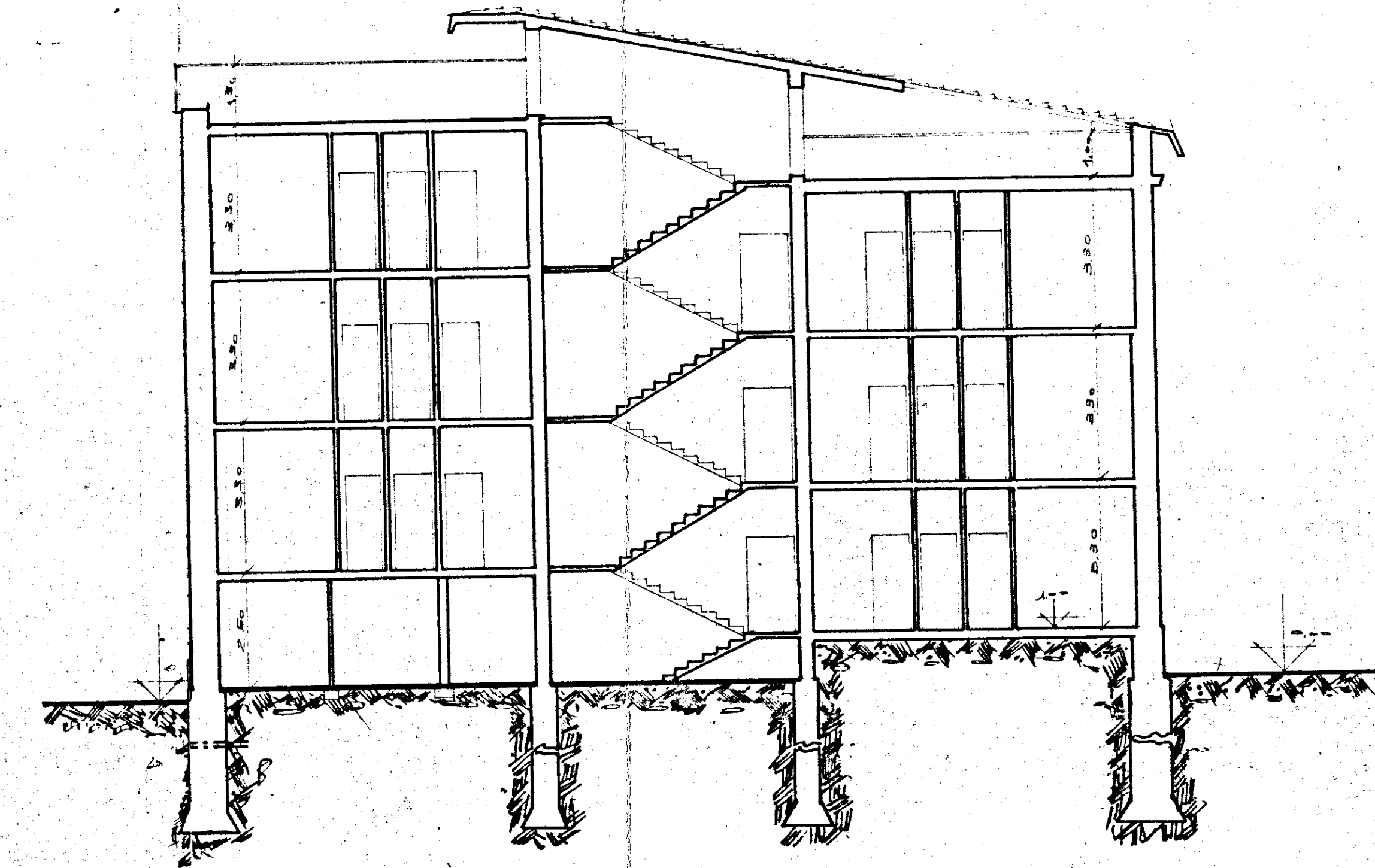
SEZIONE LONGITUDINALE
