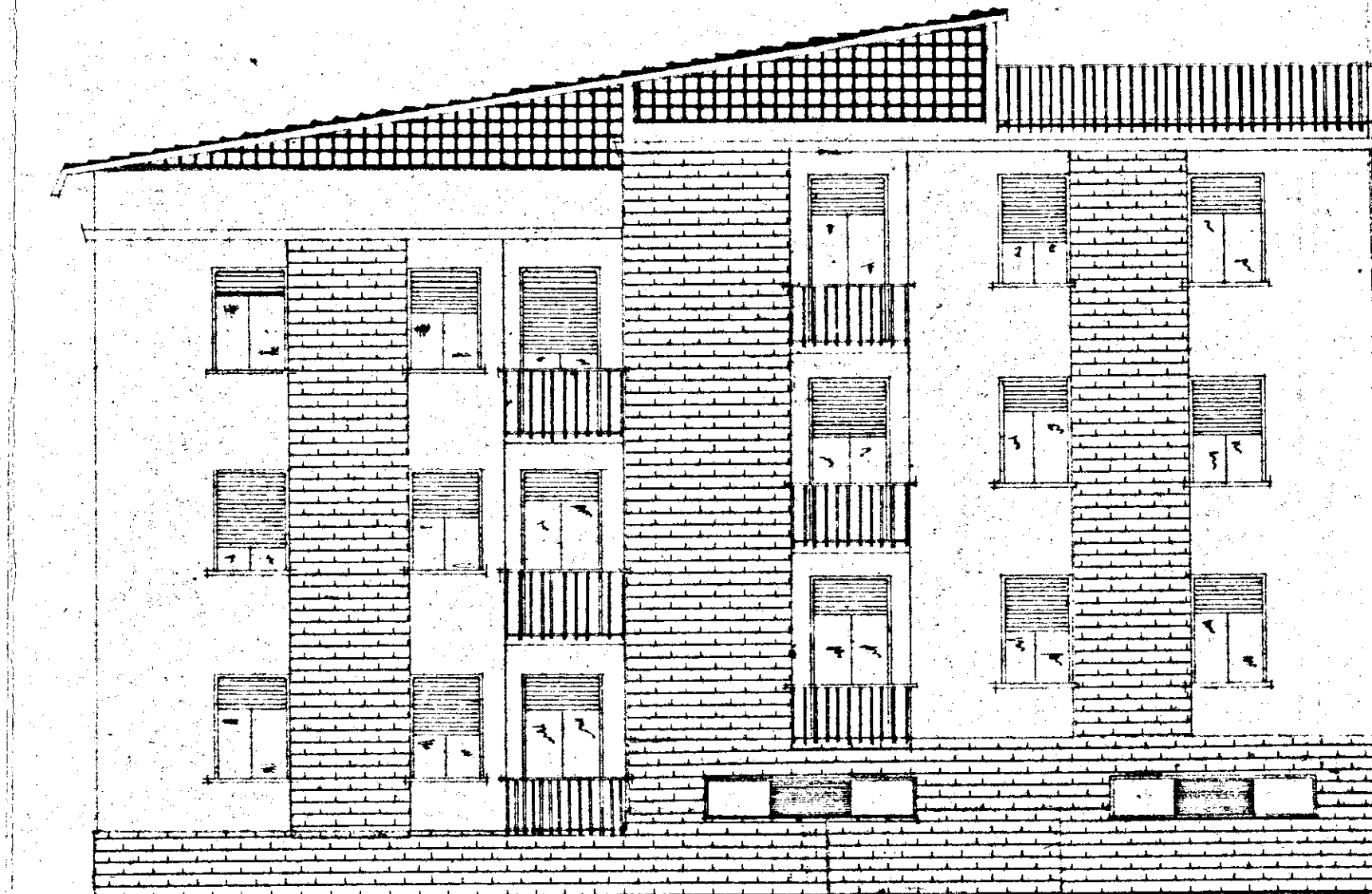
PROSPETTO POSTERIORE
