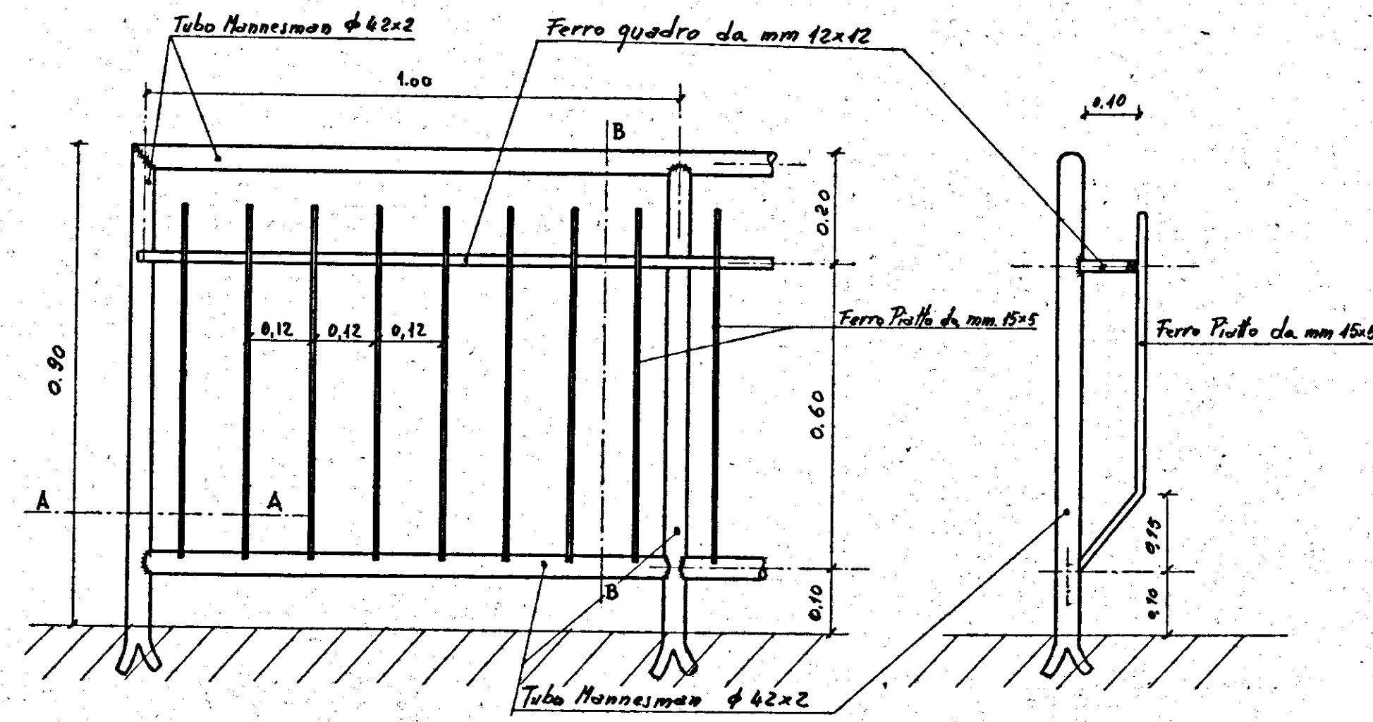
SEZ. AA SCALA 1:1
