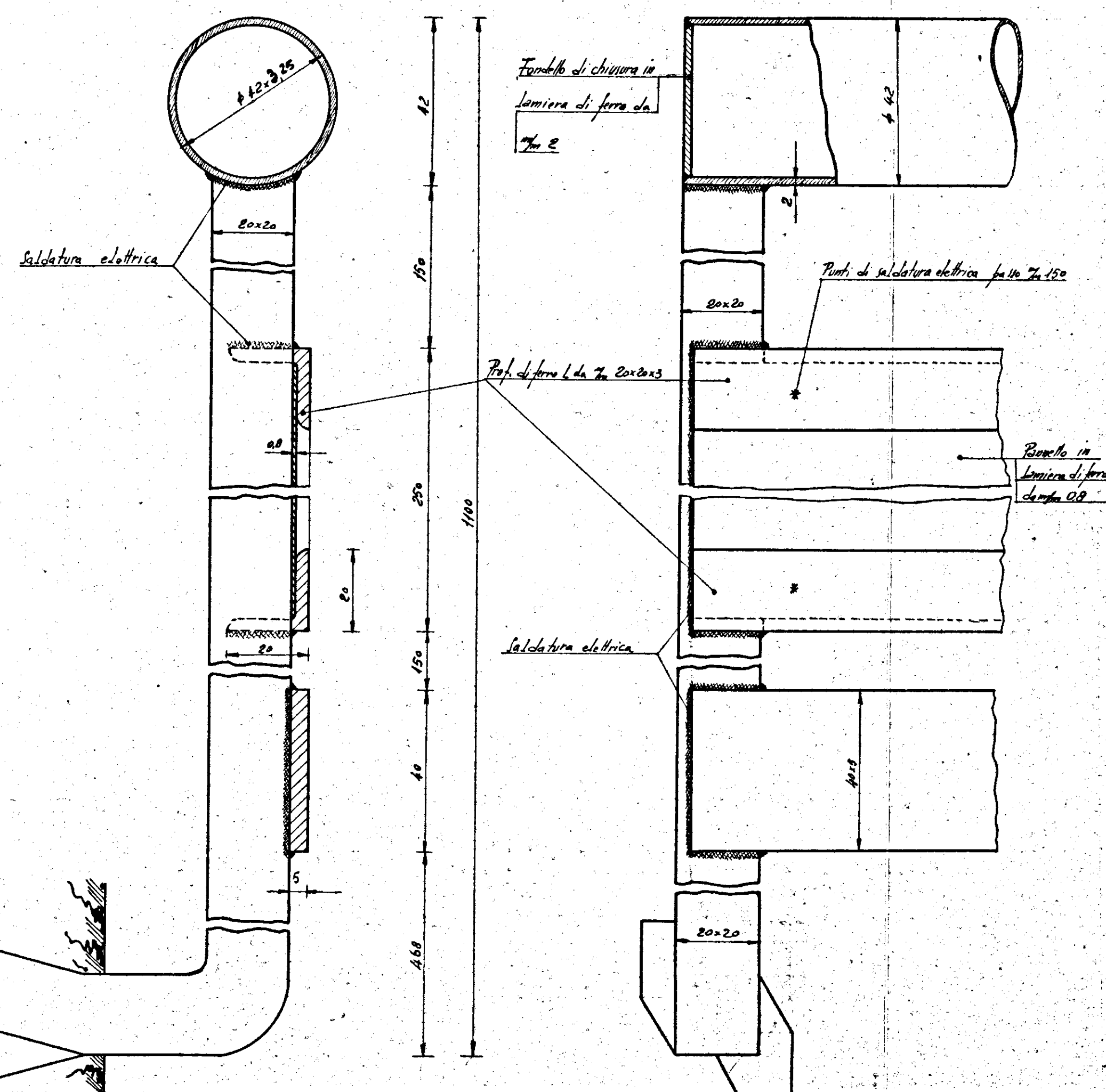
PARTICOLARE MONTANTE - SCALA 1:1
