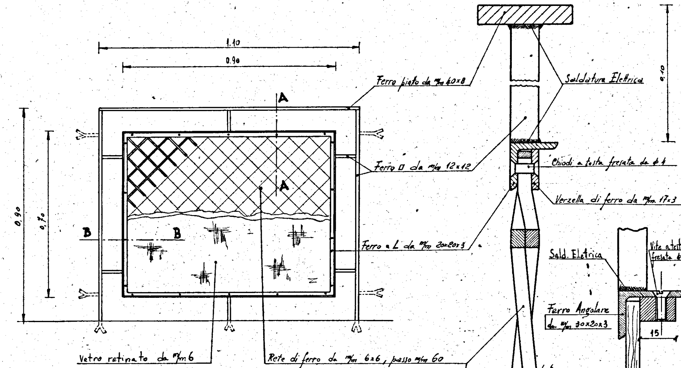
RINGHIERA PER BALCONI E VERANDE SCALA 1:10
