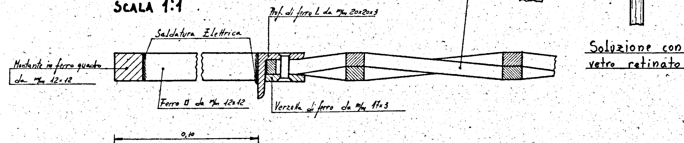
SEZ. BB SCALA 1:1
