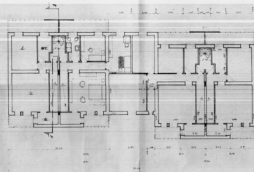
PIANTA PRIMO PIANO
